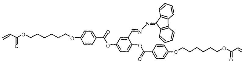
Compound 1r
