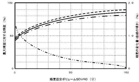
(a)特性曲線
