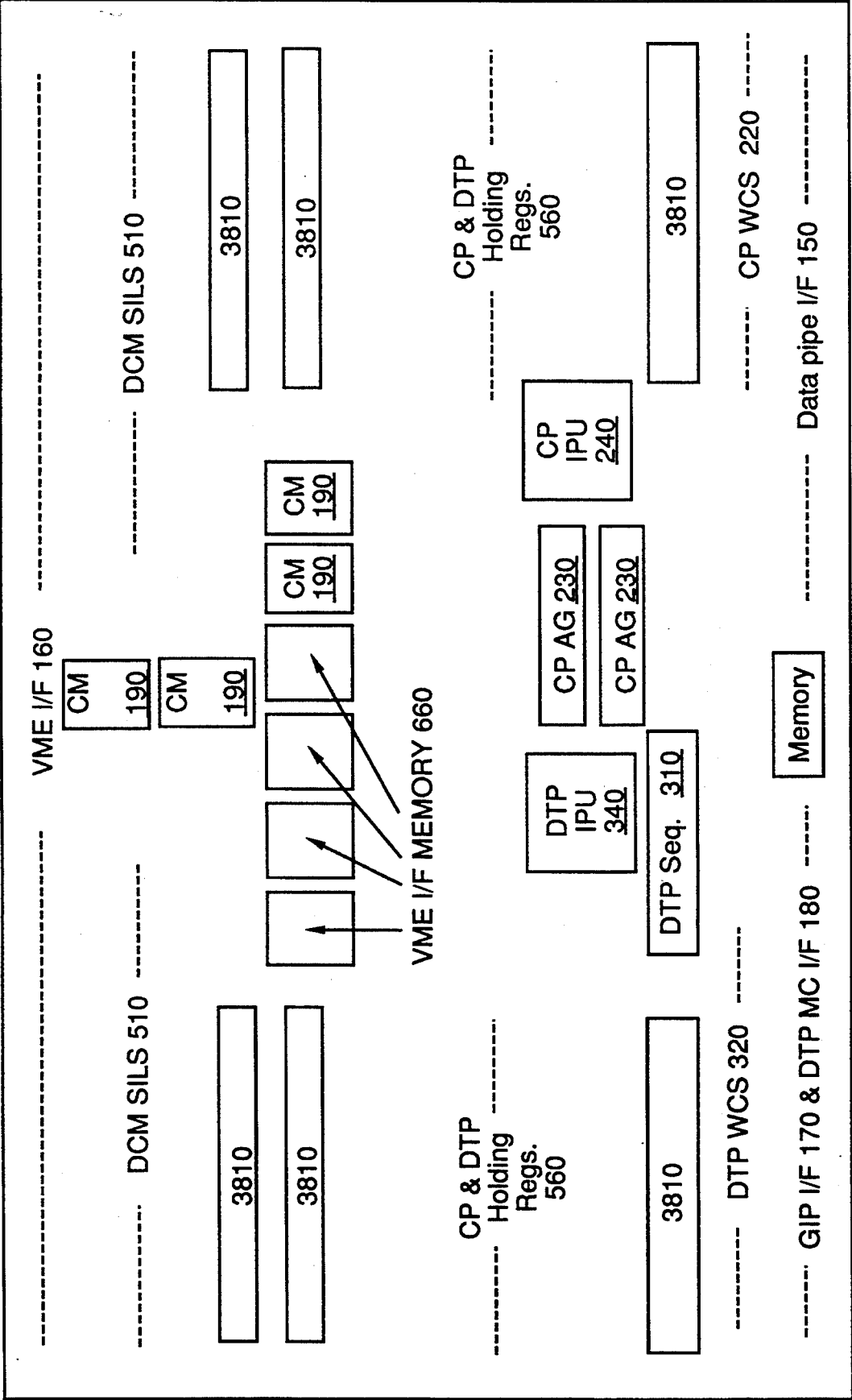
Fig. 38A
