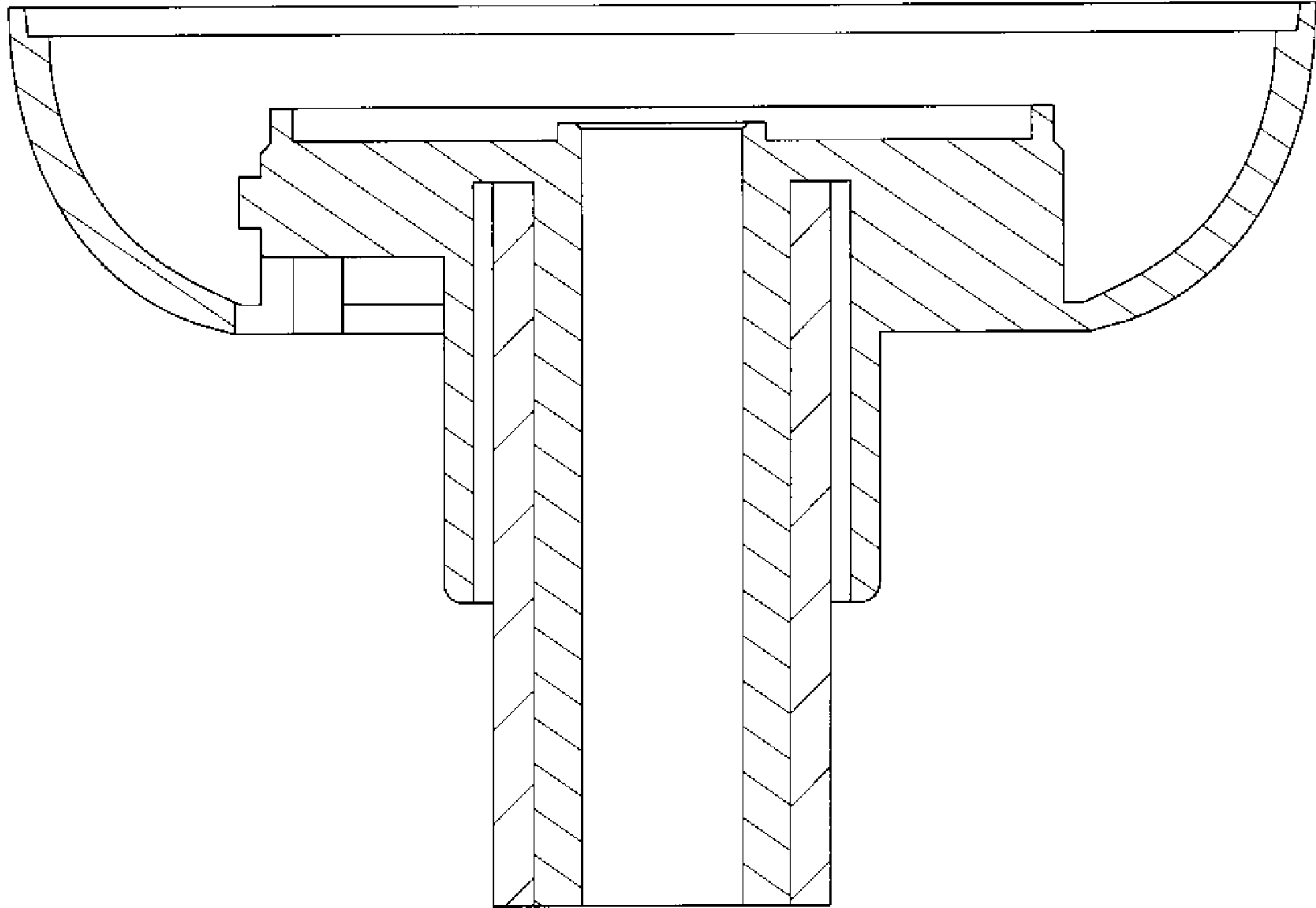
【A-A部之B-B線放大剖視圖】
