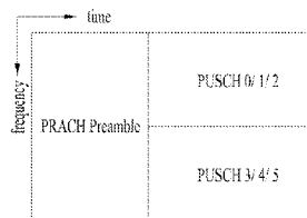
(d) FDM/CDM
