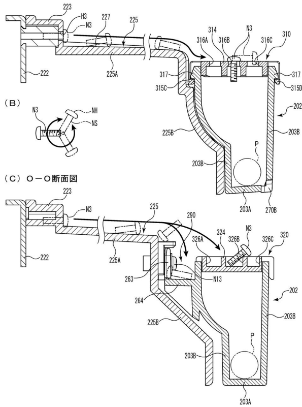
(A) N-N断面図
