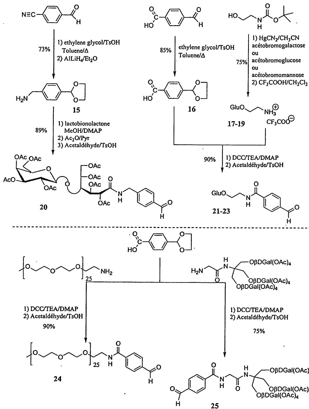
Figure 3 : synthèse des têtes polaires non ioniques
