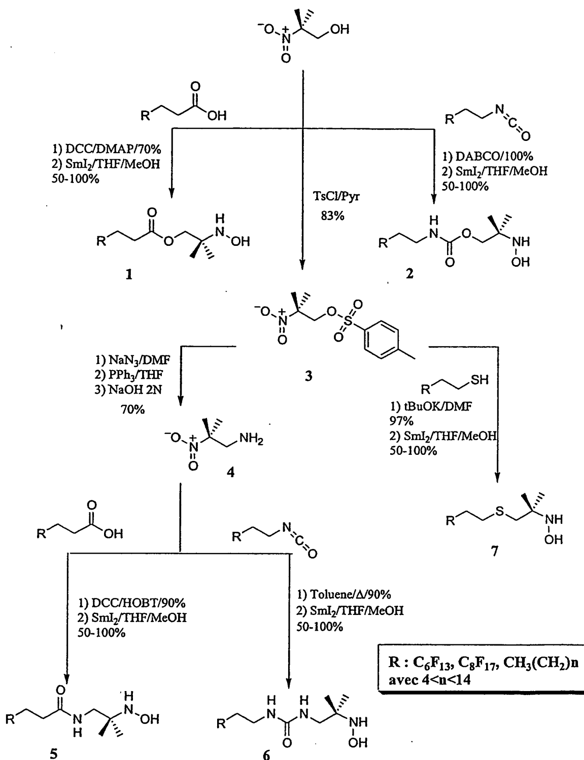
Figure 1 : synthèse des parties hydrophobes monocaténaires hydro et perfluorocarbonées
