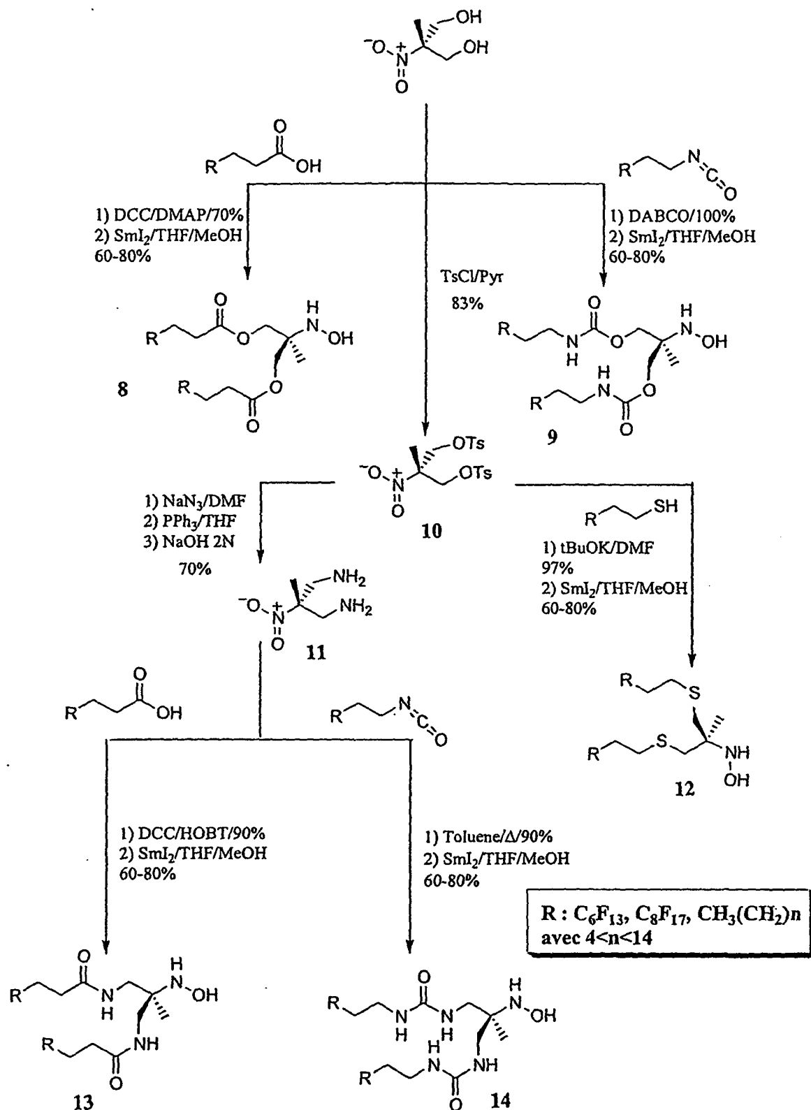
Figure 2 : synthèse des parties hydrophobes bicaténaires hydro et perfluorocarbonées
