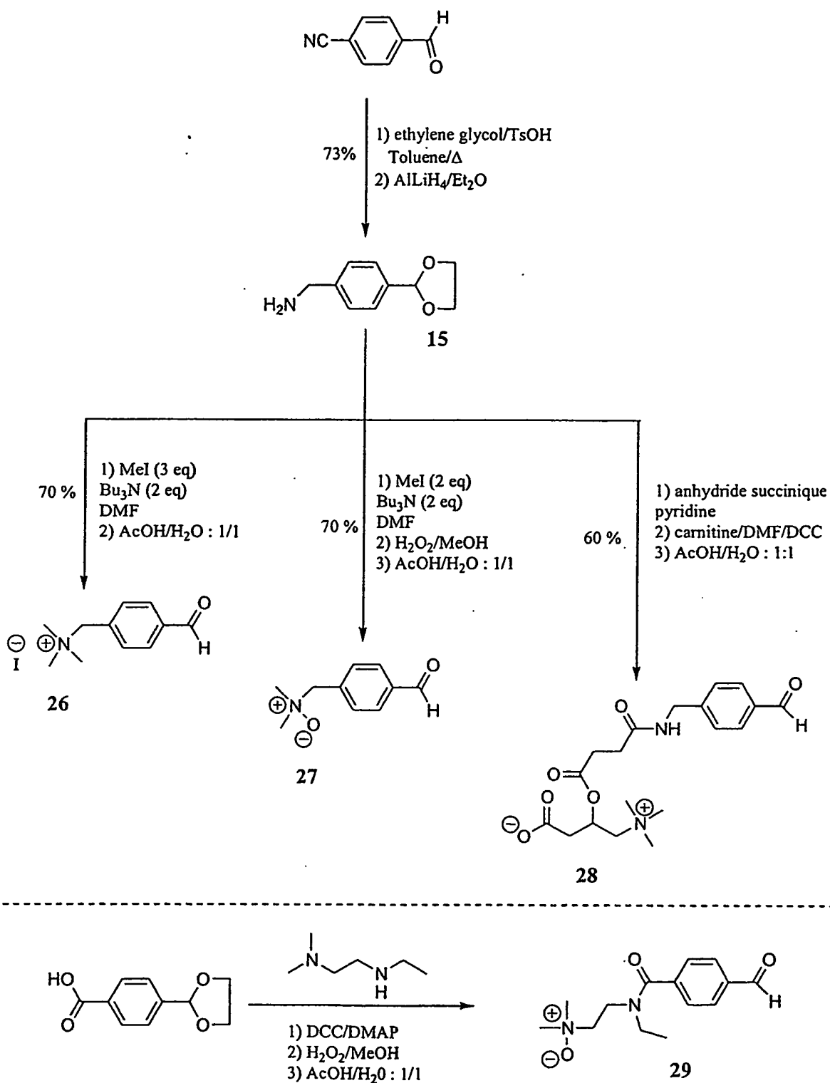
Figure 4 : synthèse des têtes polaires ioniques
