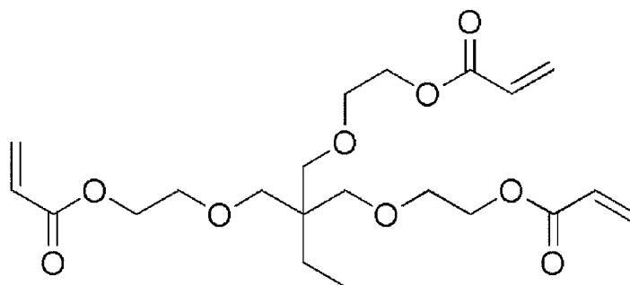
Polymerizable Monomer 1
