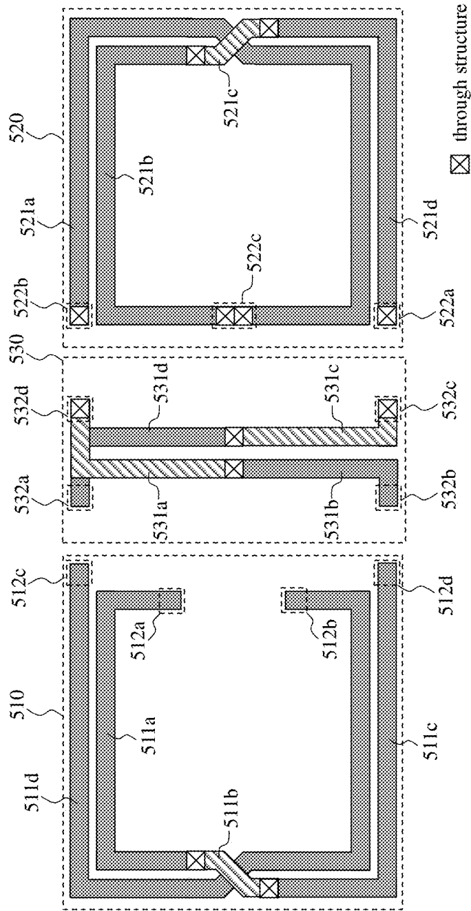
Fig. 5B
