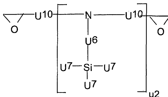
(Xa)
