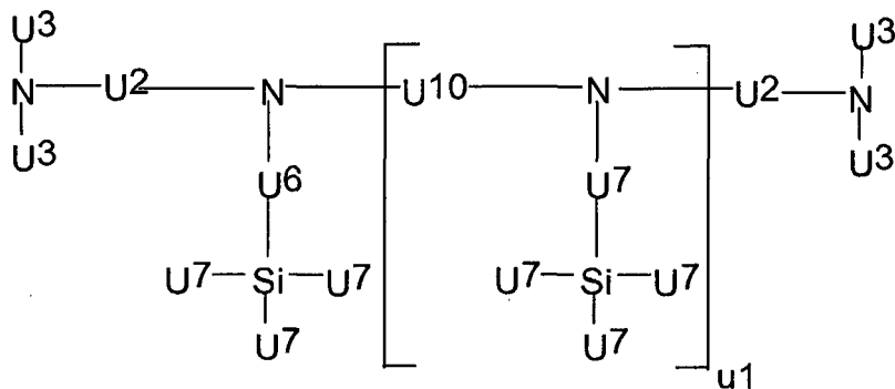
(IXd)
