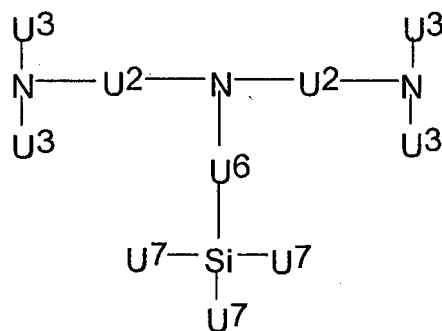
(IXb)
