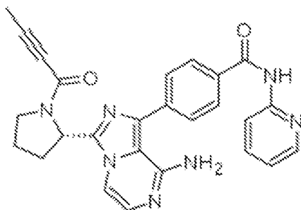
Acalabrutinib
