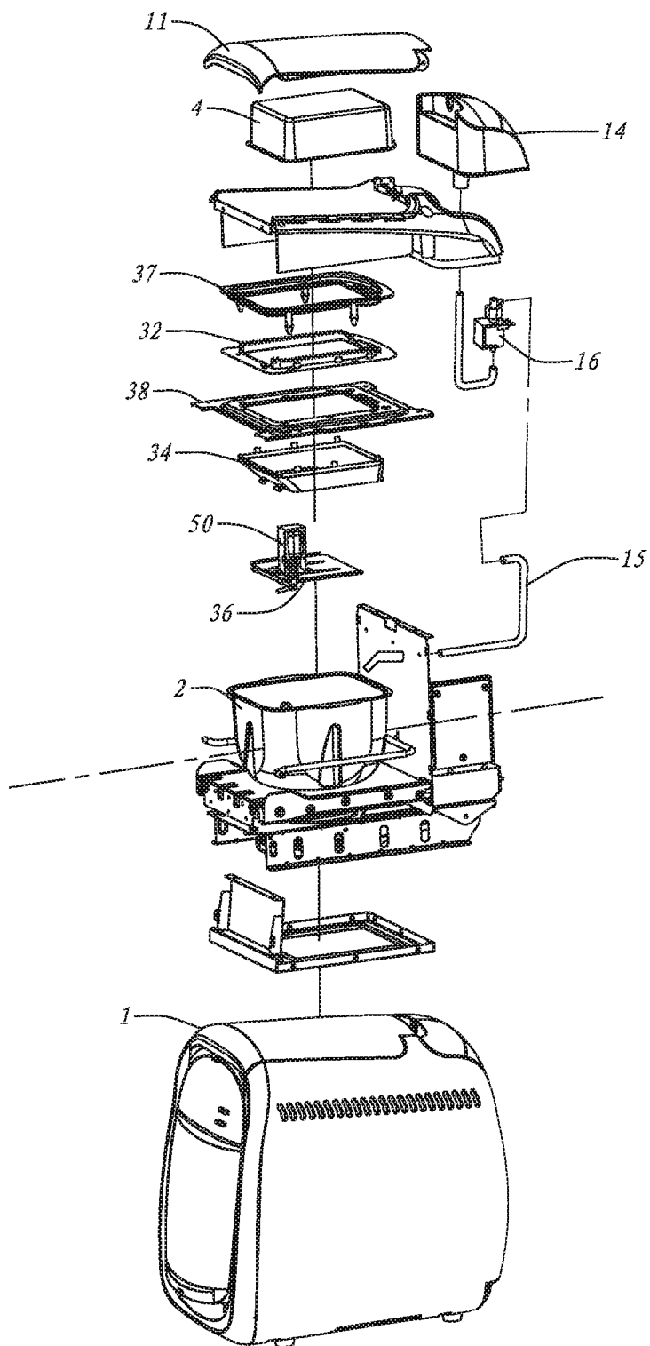
FIG. 14
