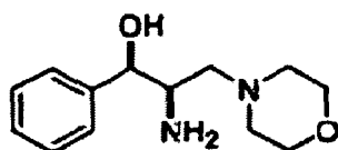
40 2 HCl L-thréo
