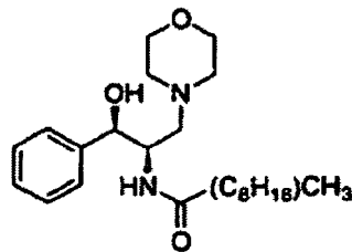
D-thréo-PDMP
