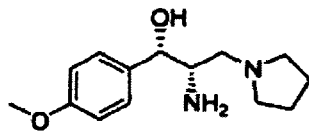
DI-thréo
