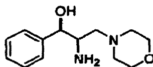
2 HCl D-thréo
