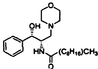
L-thréo-PDMP
