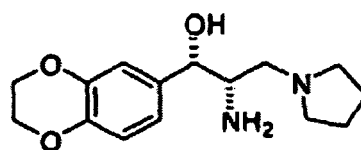
DL-thréo
