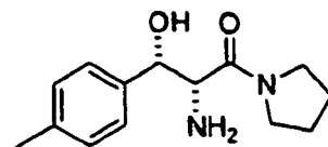
HCl DL-threo
