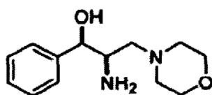
25 2 HCl DL-thréo
