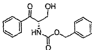
TTA 08010B
