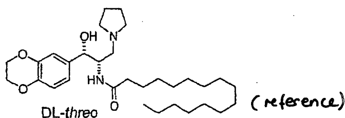
DL-threo
