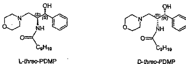
45 L-threo-PDMP
