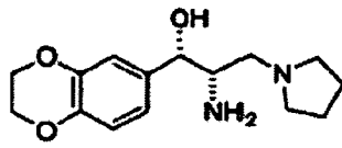
DL-thréo
