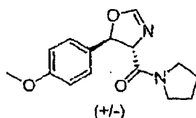
SLA 07074
