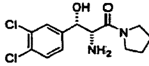
HCl DL-thréo
