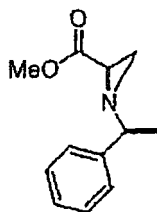
EBE 06044B
