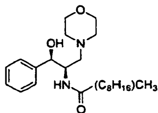
D-threo-PDMP
