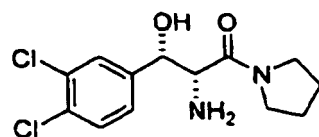
HCl DL-threo
