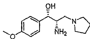
DL-threo
