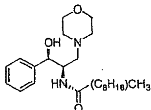
D-threo-PDMP
