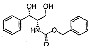
TTA 08012
