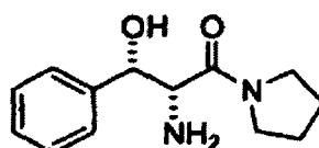
HCl DL-thréo
