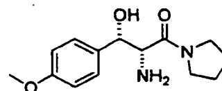
HCl DL-threo
