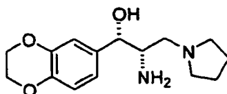
DL-threo
