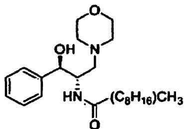
DL-érythro-PDMP
