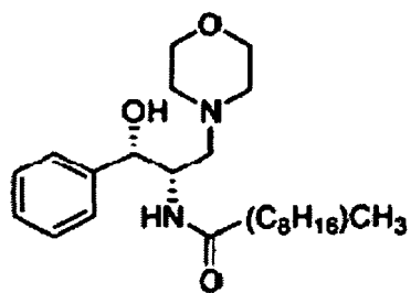
L-thréo-PDMP
