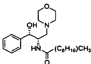
L-threo-PDMP
