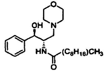
DL-érythro-PDMP
