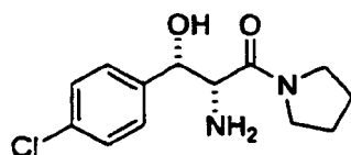
HCl DL-threo
