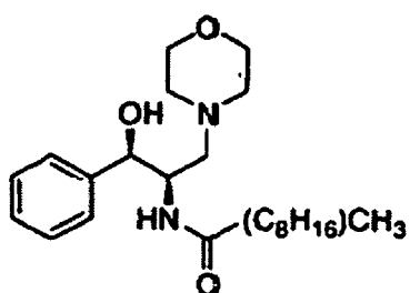
D-thréo-PDMP
