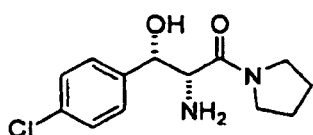
HCl DL-threo
