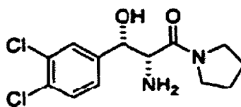
10 HCl DL-thréo
