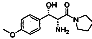
HCl DL-thréo
