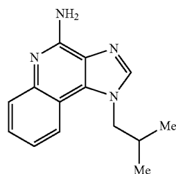
Imiquimod
