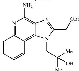
Resiquimod
