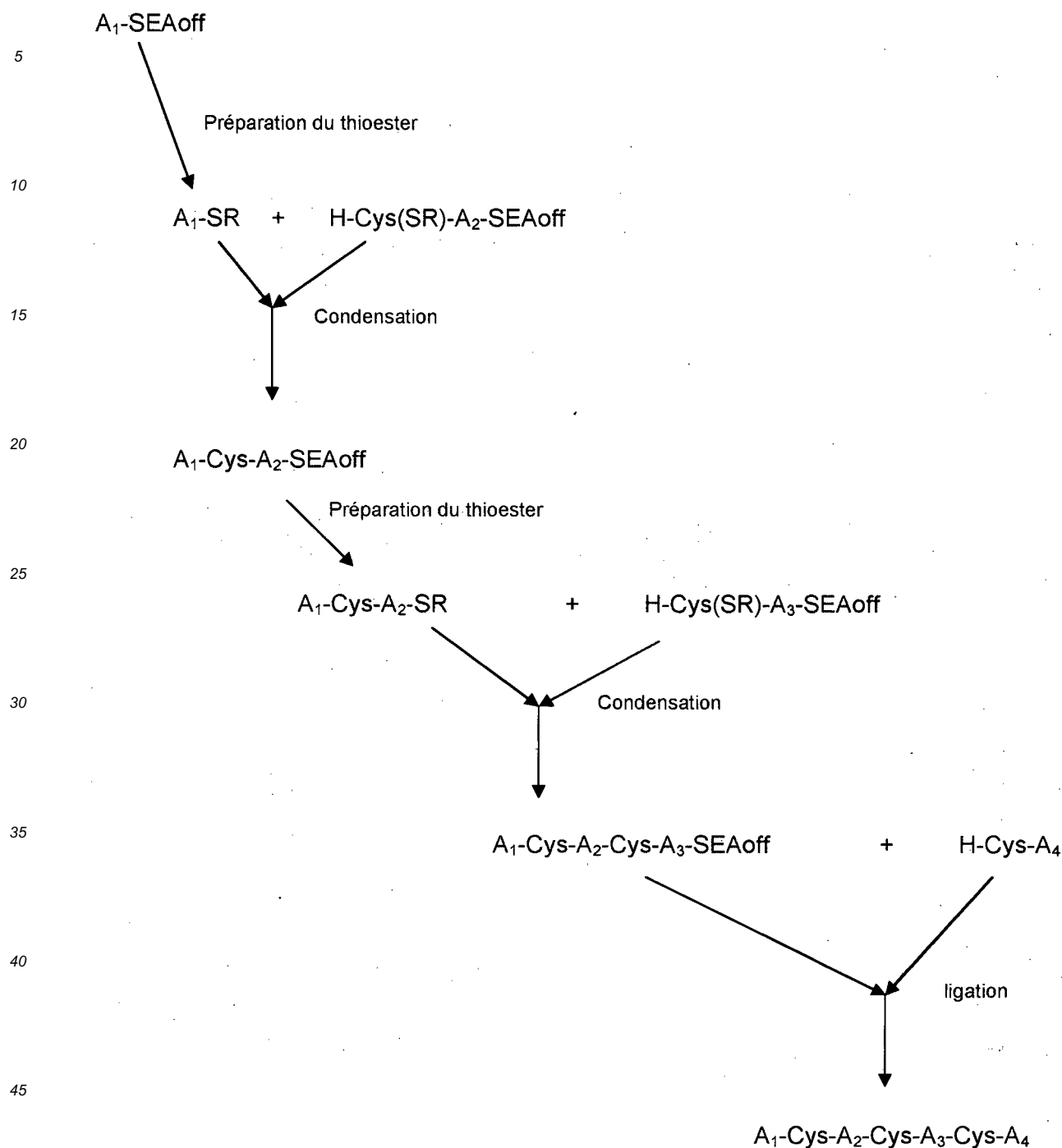
Schéma 2
