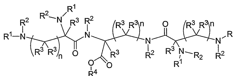
VII
