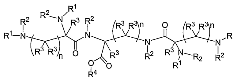
VII
