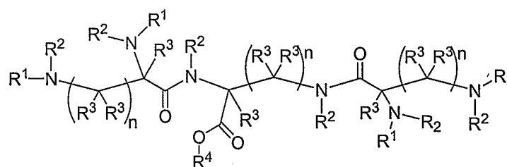
VII
