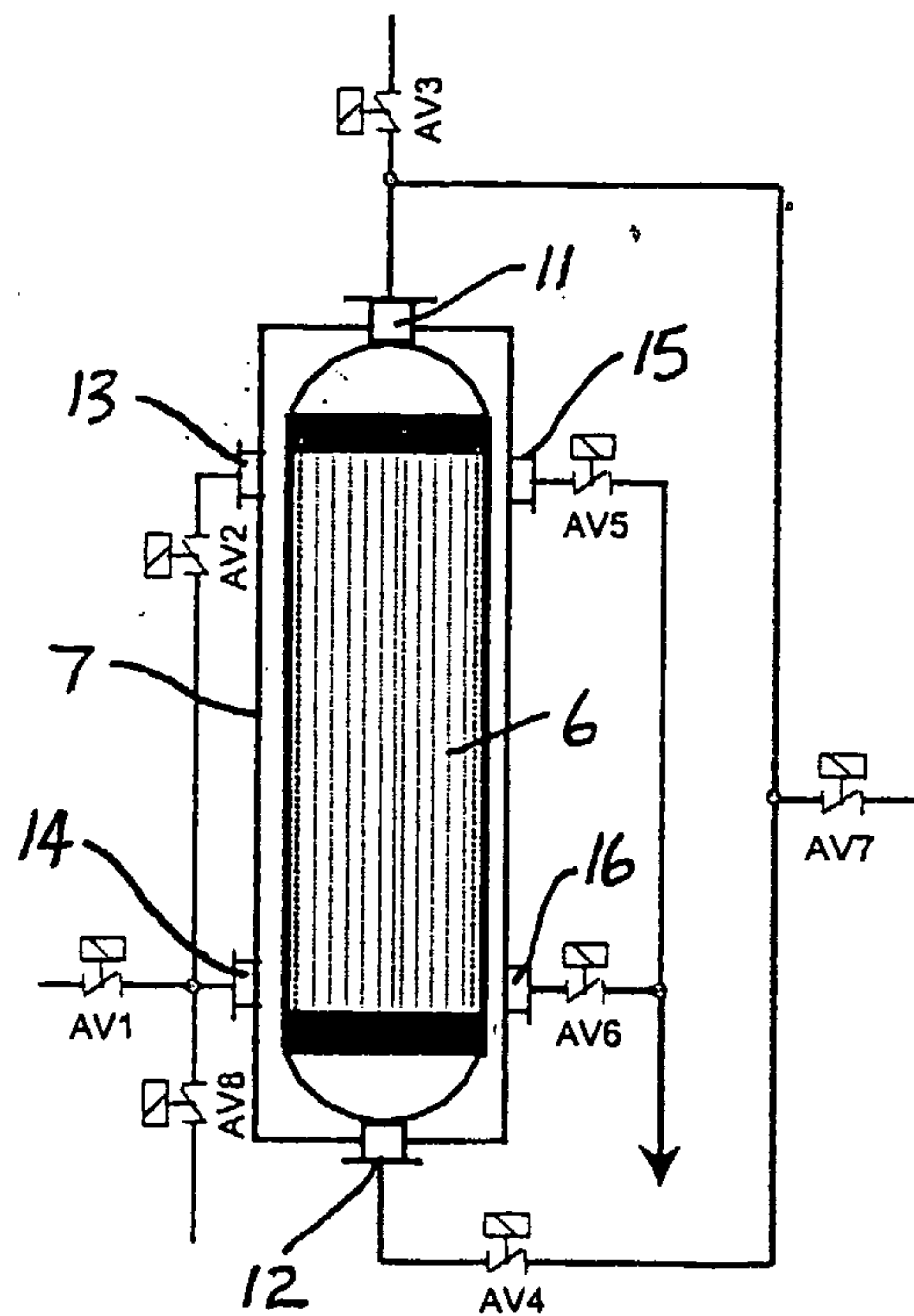
(d) Blow-out and fast drain-down
