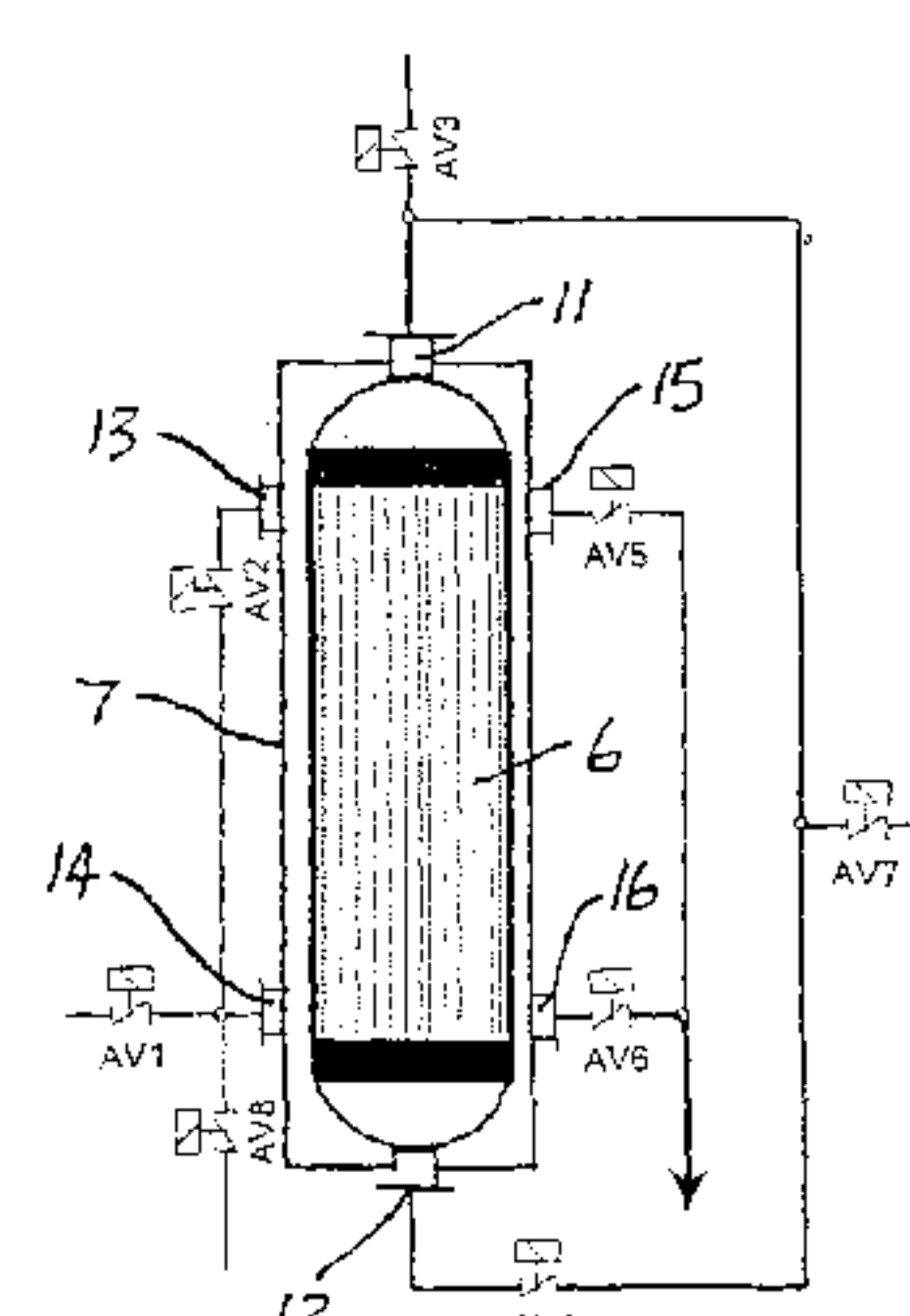
(d) Blow-out and fast drain-down
