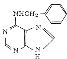
6-benzylaminopurine
