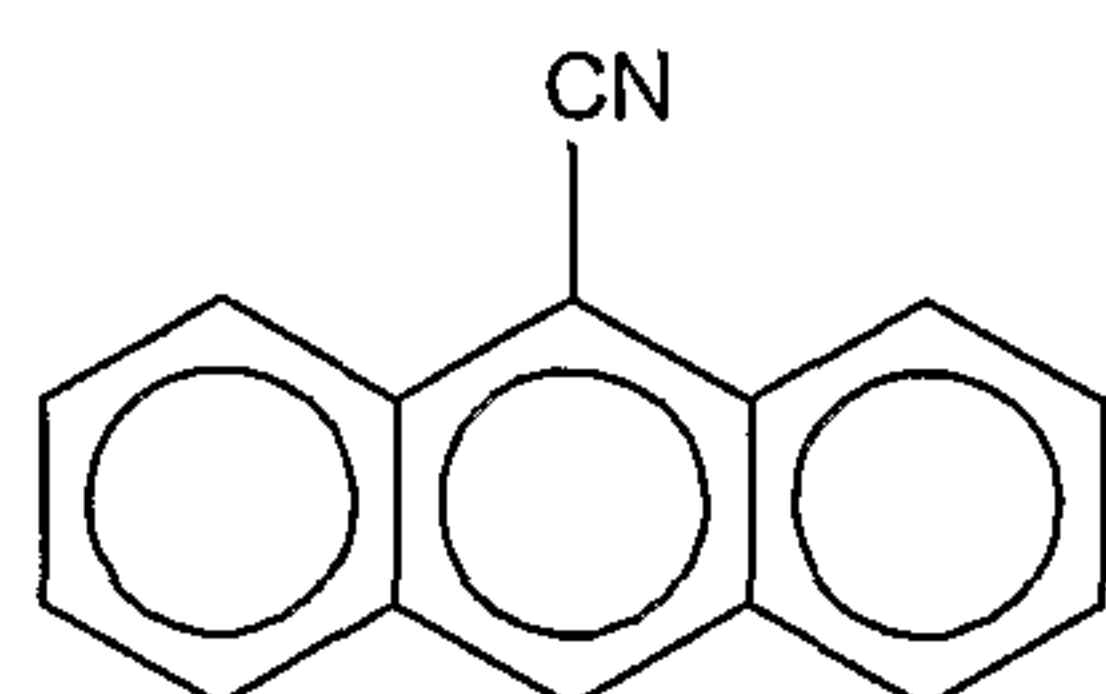
9' anthracenecarbonitrile MW = 203
