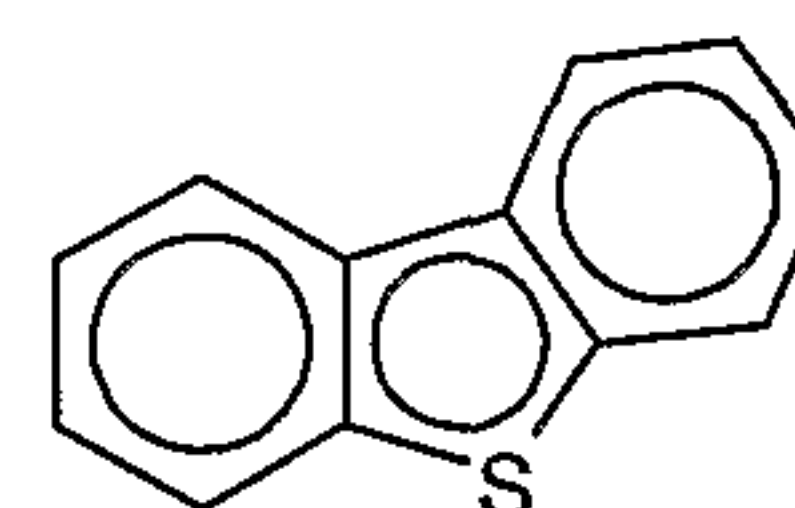
dibenzothiophene MW = 184
