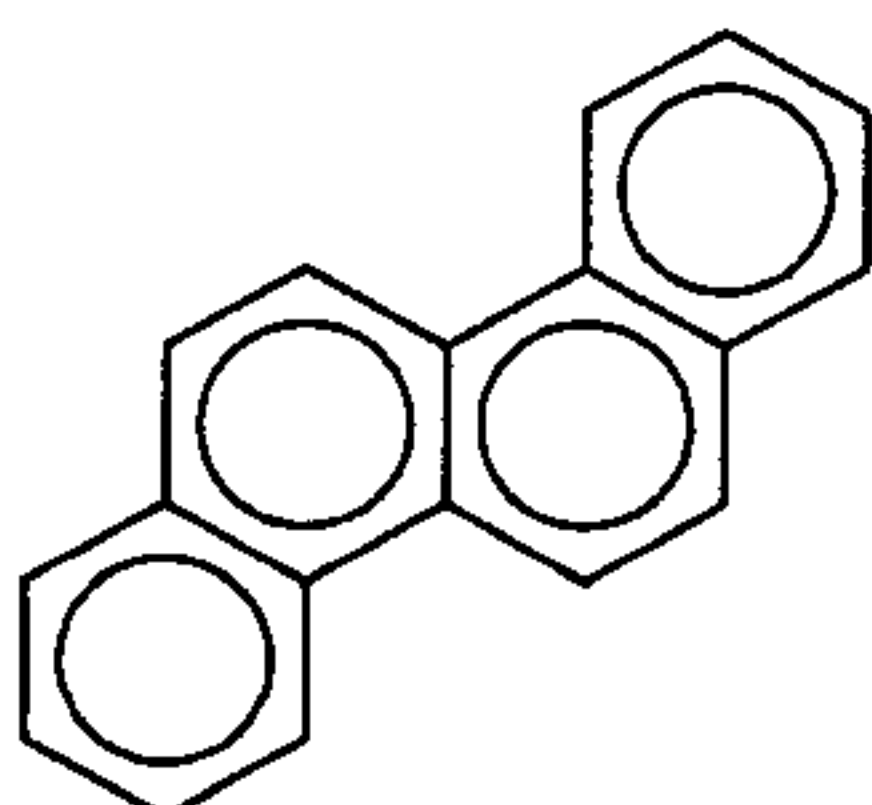
chrysene MW = 228
