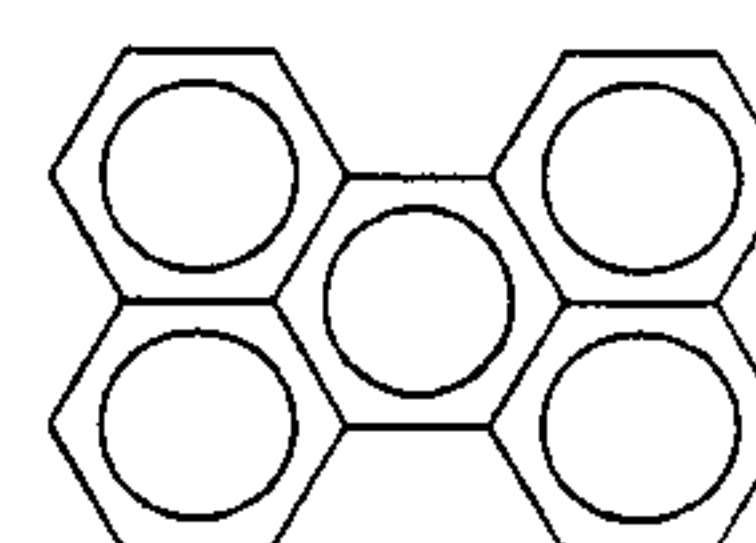
perylene MW = 252
