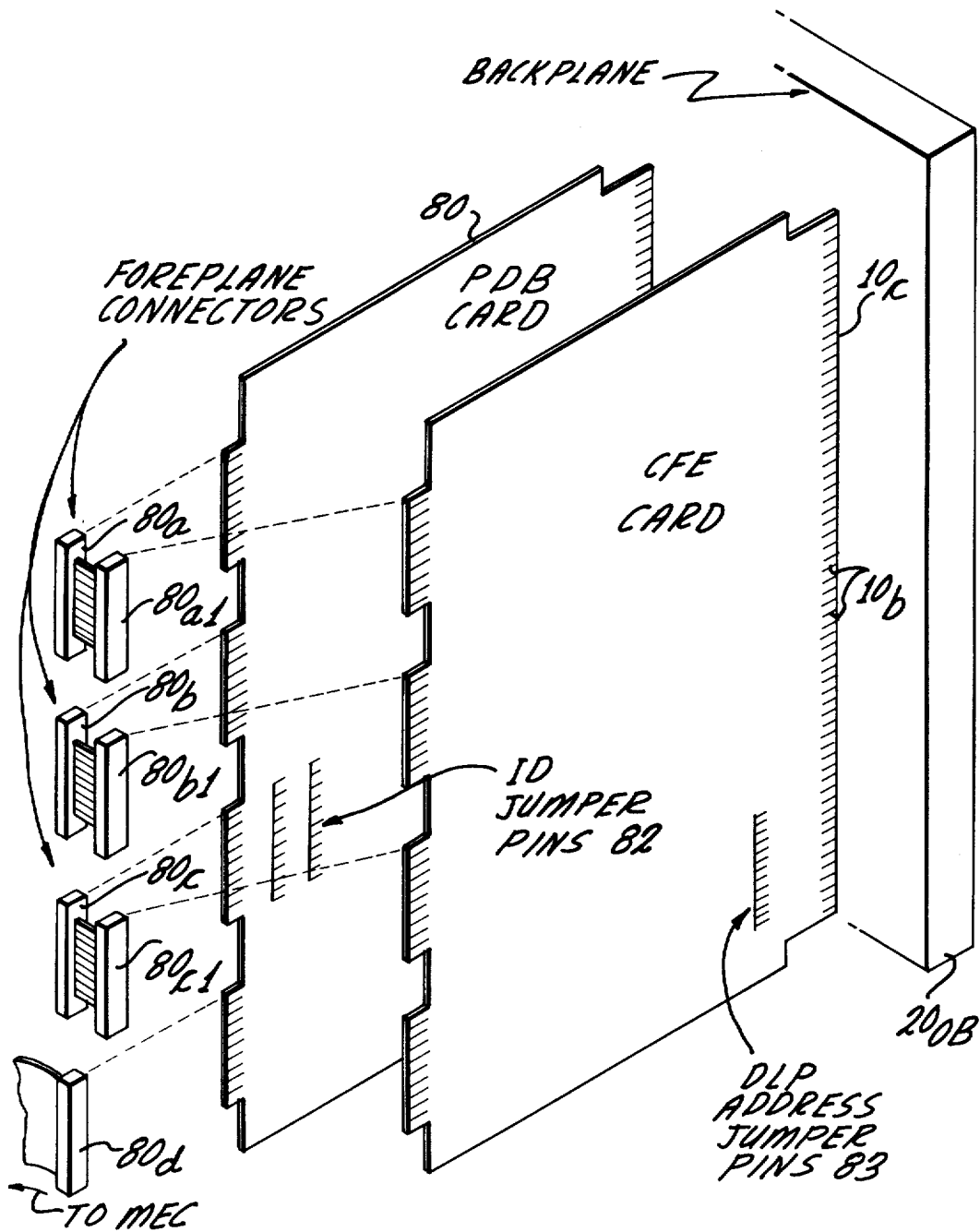
Fig. 3 DLP MODULE ASSEMBLY
