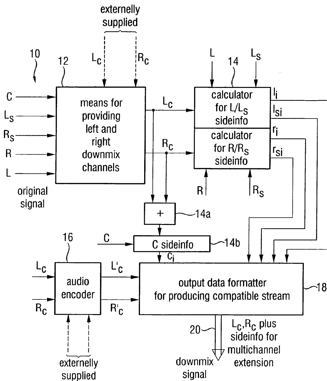
FIG 1A (Encoder)
