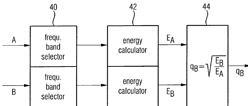
FIG 4 (encoder side)
