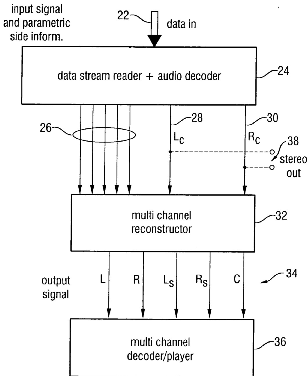
FIG 2A (Decoder)
