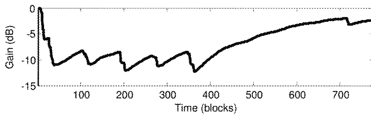
FIG. 10e e) Event-controlled DRC gain
