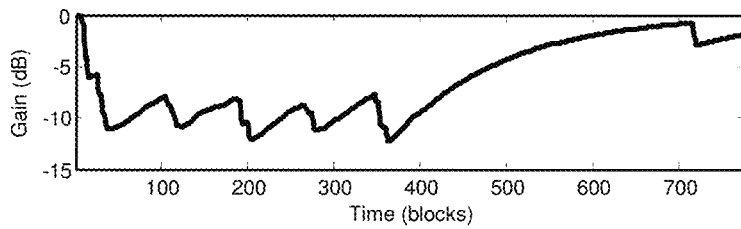
FIG. 10b b) DRC gain
