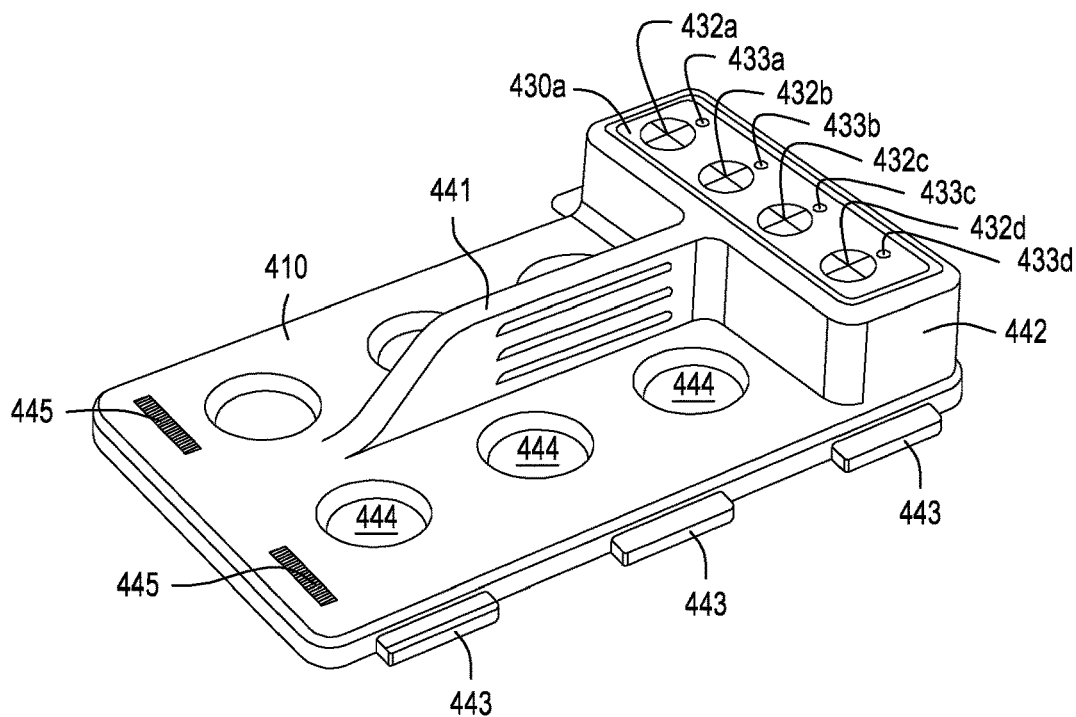
FIG. 4S
