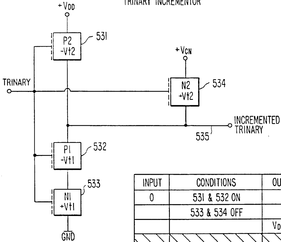
FIG. 14A. TRINARY INCREMENTOR
