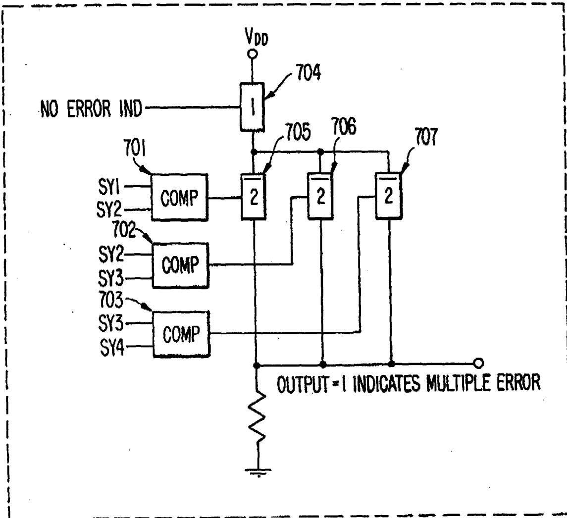
FIG. 13. MULTIPLE ERROR DETECTOR 700
