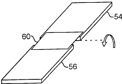
FLAT NITINOL HINGE FIG. 4A
