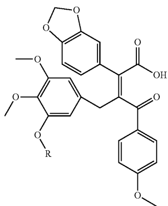
16 R 3 = CH 3 (PD156707) 17 R = CH 2 CH 2 CH 2 SO 3 H
