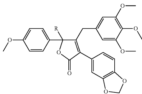
18 R = OCH 2 CH 2 CH 2 SO 3 H 19 R = OCONHCH 2 CO 2 C 2 H 5
