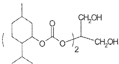
(IIe)
