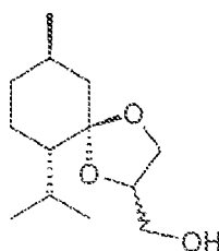
(1aa)
