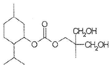
(IIf)
