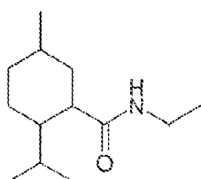
(IVa)
