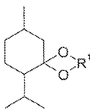
(Ia)
