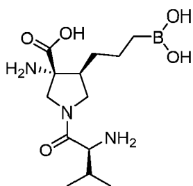
Valine AUC = 13701
