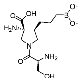
Serine AUC = 14784
