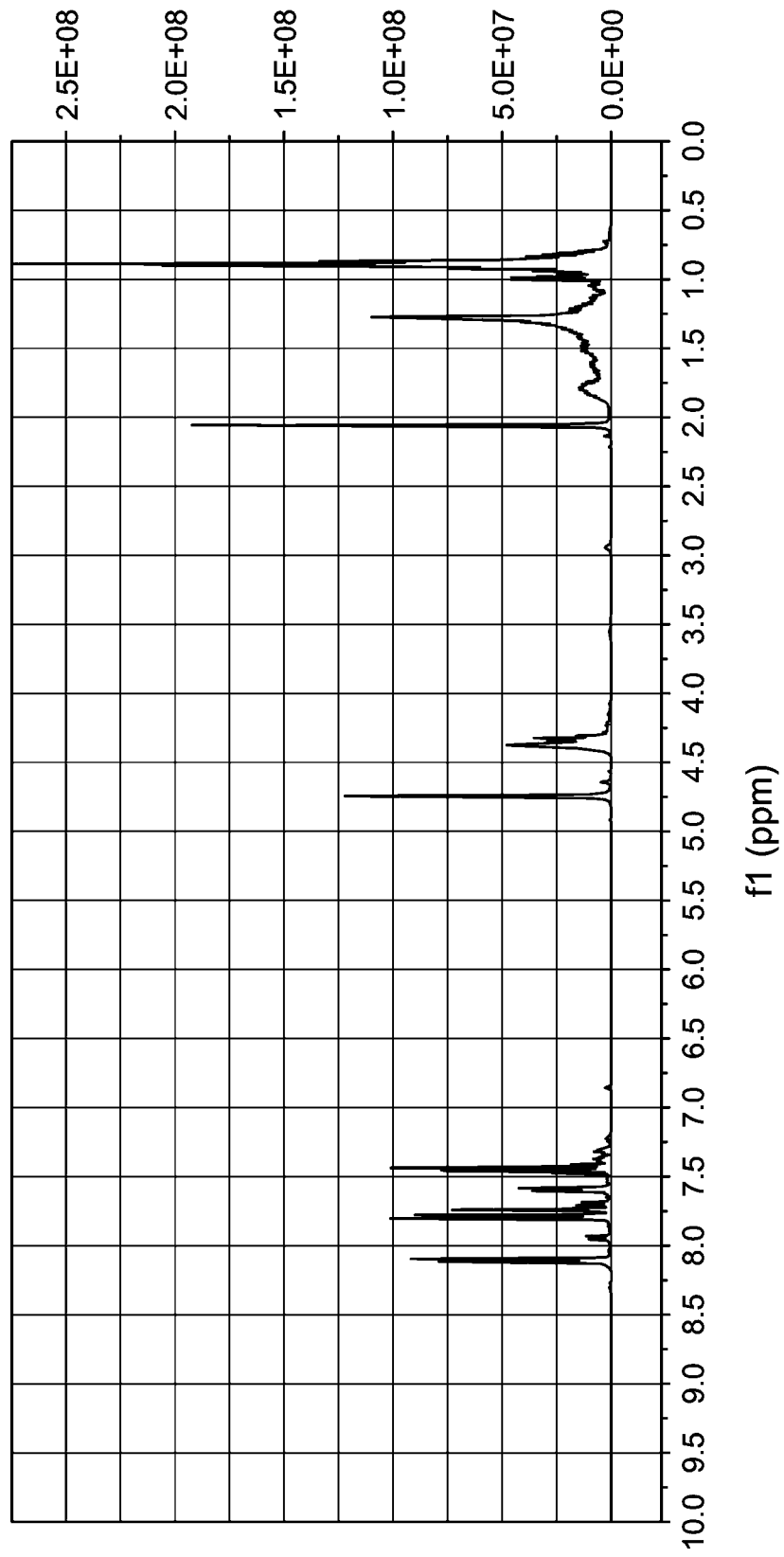
f1 (ppm) FIG. 2
