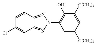
TINUVIN 327 (RTM)
