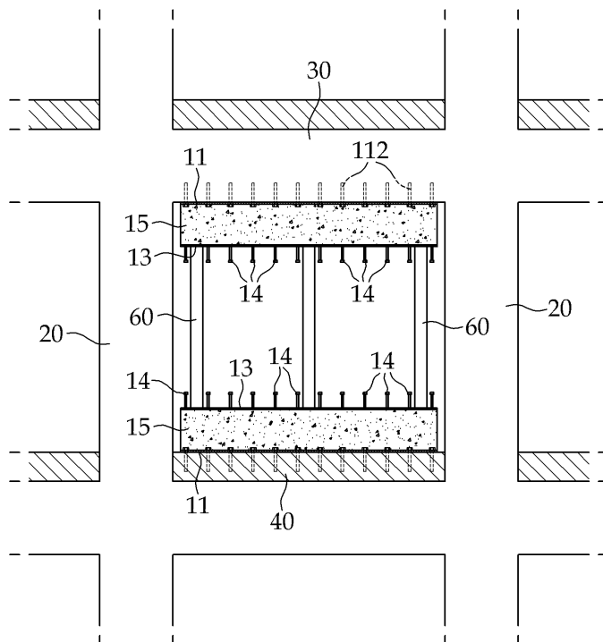
도면6
