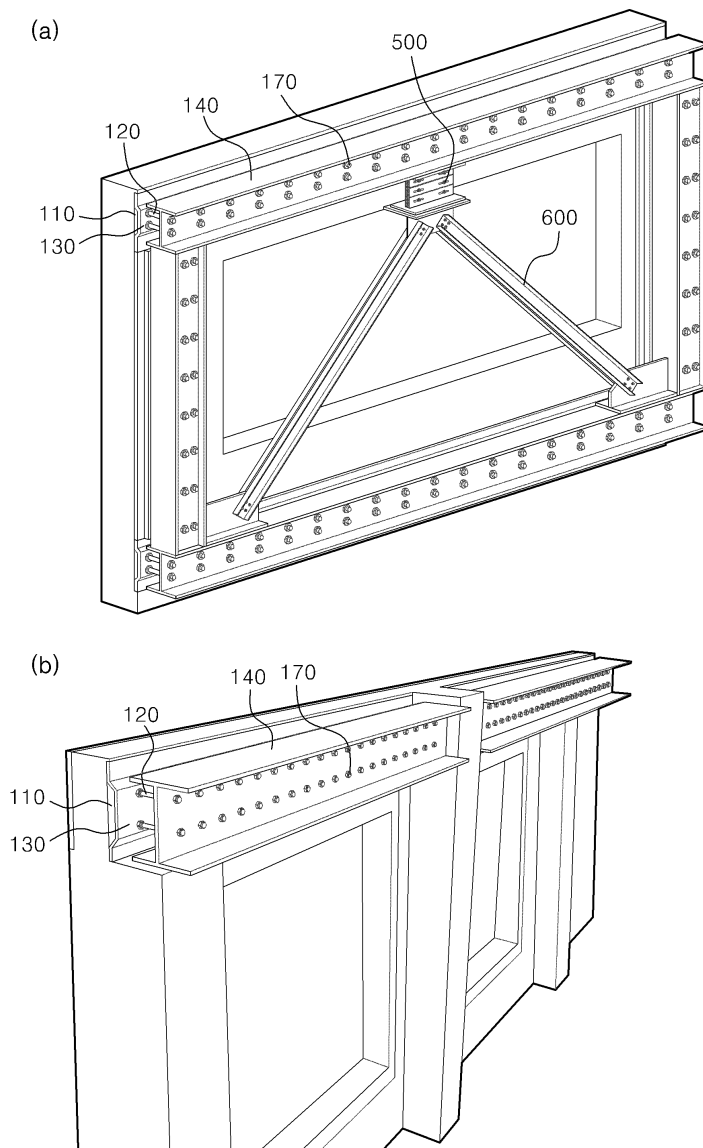
도면9
