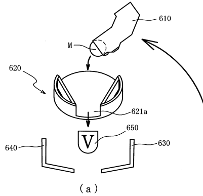
V振り分け装置が中央位置で停止しV通過
