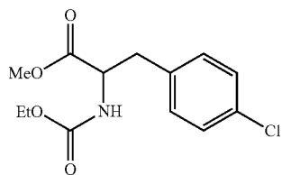
Step 2: Methyl 3-(4-chlorophenyl)-2-(ethoxycarbonylamino)propanoate
