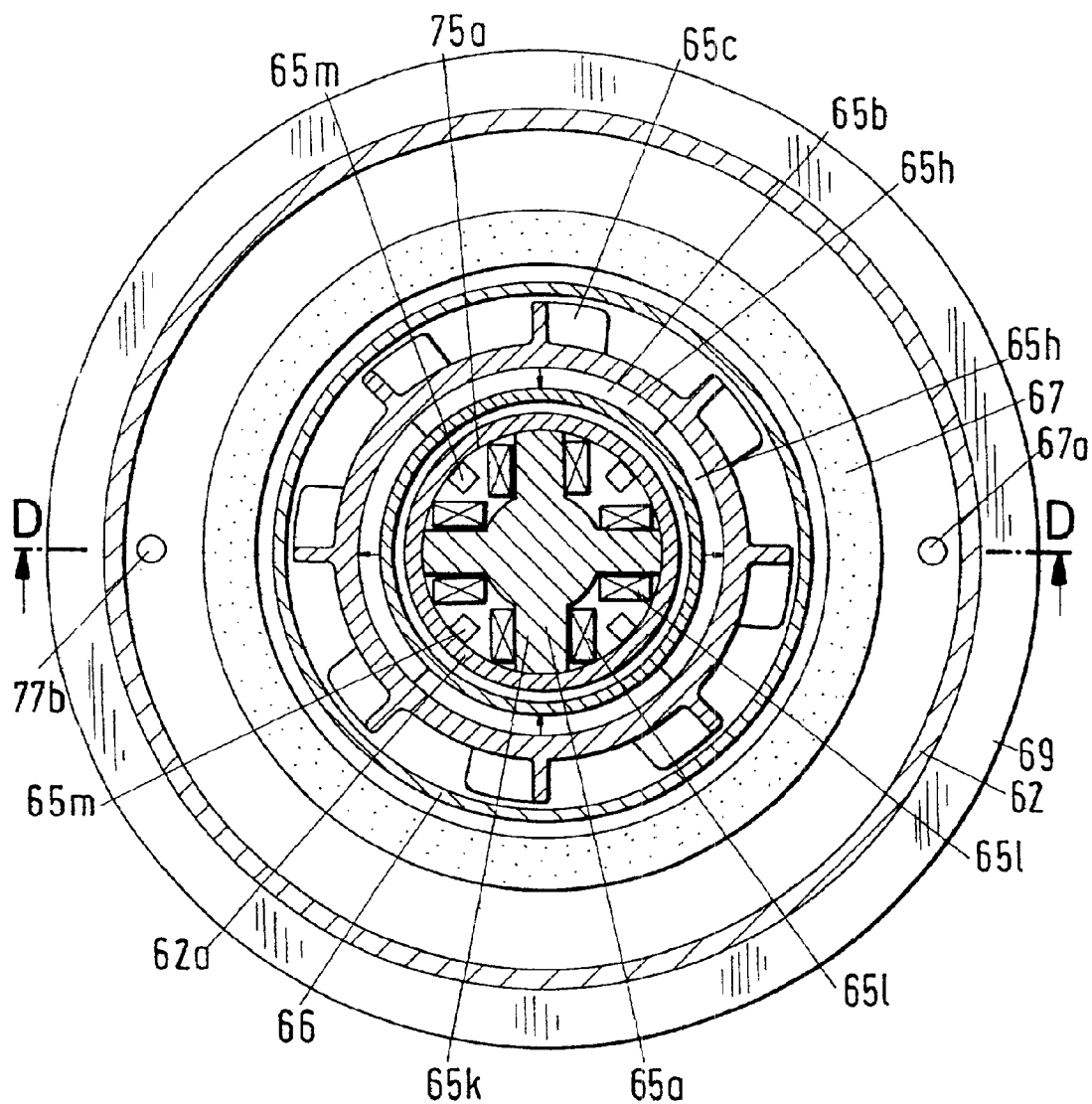
Fig. 8 C-C
