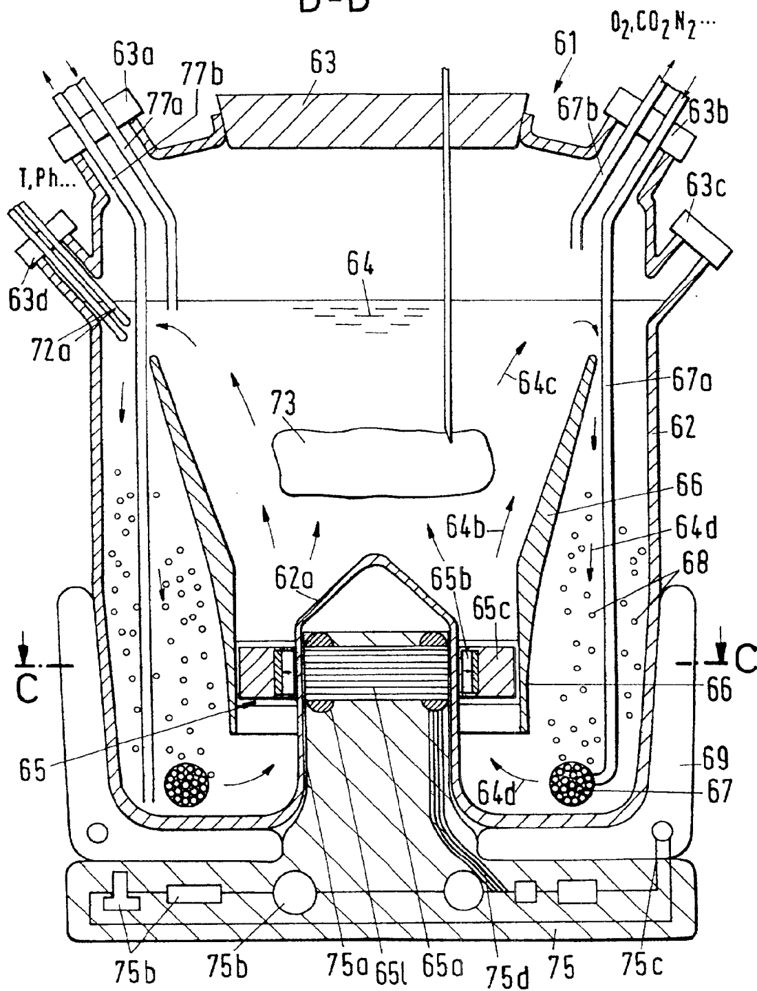
Fig. 7 D-D
