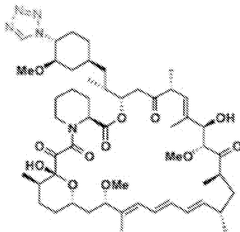
Zotarolimus (ABT-578)
