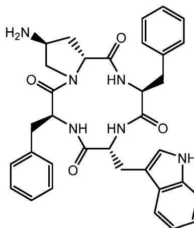
cyclo [Phe- trans -D-Amp-Phe-D-Trp],
