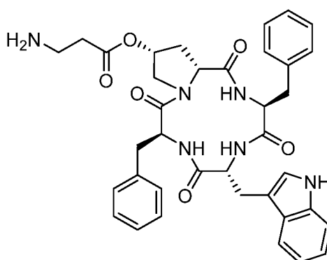
cyclo [Phe- cis -D-Hyp(β-Ala) 2 -Phe-D-Trp];
