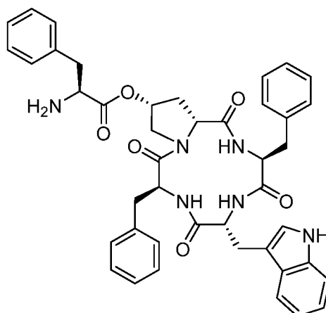
cyclo [Phe- cis -D-Hyp(Phe) 2 -Phe-D-Trp];
