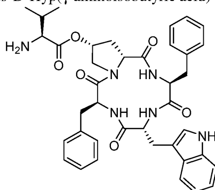
cyclo [Phe- cis -D-Hyp(Val) 2 -Phe-D-Trp];
