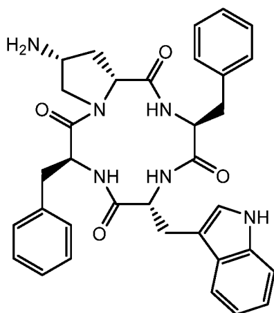
cyclo [Phe- cis -D-Amp-Phe-D-Trp],
