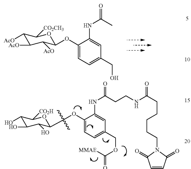
Scheme 2a
