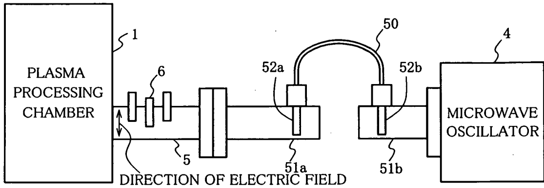
(a)TE MODE
