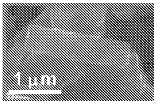
nanorod
