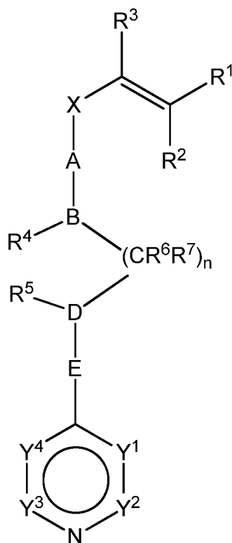
Formula (I a)
