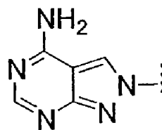
N8-(7-deaza-8-aza-A)
