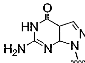
N9-(7-deaza-8-aza-G)
