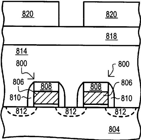
FIG. 8G BACKGROUND ART
