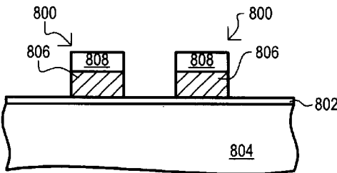
FIG. 8A BACKGROUND ART
