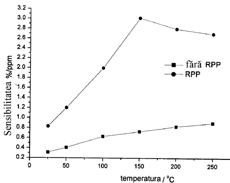
Fig. 3. Dependența sensibilității senzorului \text{Cu}_2\text{O} de temperatura de operare la gazul toxic 1,5 ppm \text{NO}_2 .
