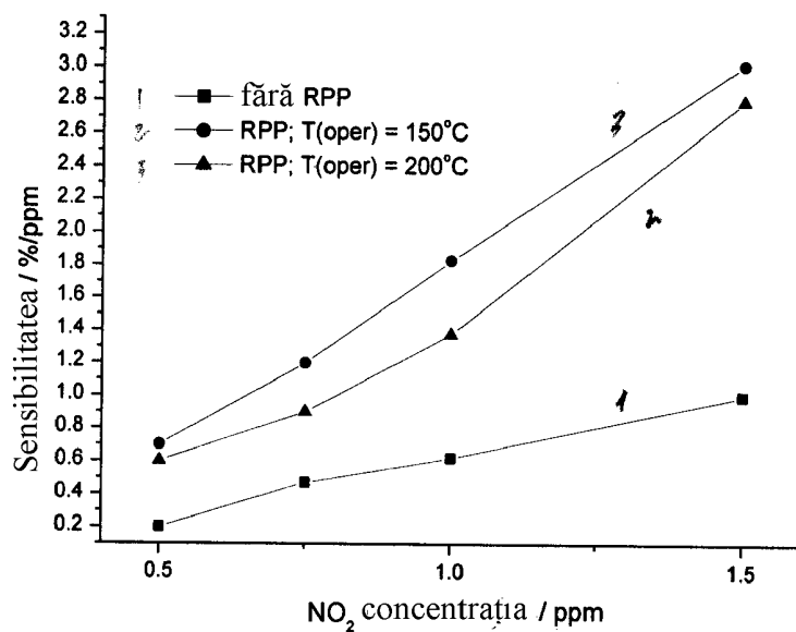
Fig. 4. Dependența sensibilității senzorului \text{Cu}_2\text{O} de concentrația gazului toxic \text{NO}_2 la diferite temperaturi de operare. Proba 1 – fără procesarea fototermică rapidă, 2,3 – cu procesarea fototermică rapidă, t^\circ = 350^\circ\text{C} , t = 7\text{s} .
