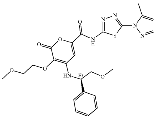
(R)-4-((2-methoxy-1-phenylethyl)amino)-3-(2-methoxyethoxy)-N-(5-(5-methyl-1H-pyrazol-1-yl)-1,3,4-thiadiazol-2-yl)-2-oxo-2H-pyran-6-carboxamide
