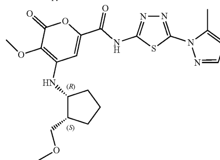
Compound 80* 3-methoxy-4-(((1R,2S)-2-(methoxymethyl)cyclopentyl)amino)-N-(5-(5-methyl-1H-pyrazol-1-yl)-1,3,4-thiadiazol-2-yl)-2-oxo-2H-pyran-6-carboxamide
