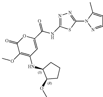
3-methoxy-4-(((1S,2R)-2-methoxycyclopentyl)amino)-N-(5-(5-methyl-1H-pyrazol-1-yl)-1,3,4-thiadiazol-2-yl)-2-oxo-2H-pyran-6-carboxamide
