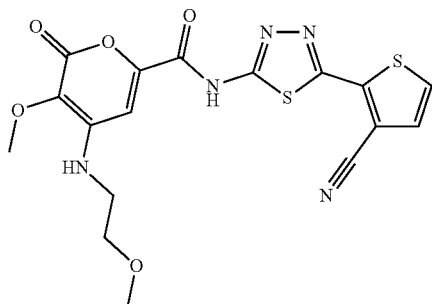
N-(5-(3-cyanothiophen-2-yl)-1,3,4-thiadiazol-2-yl)-3-methoxy-4-((2-methoxyethyl)amino)-2-oxo-2H-pyran-6-carboxamide
