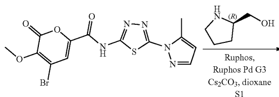
Compound 173* 4-(((1R,2S)-2-(2,2-difluoroethoxy)cyclobutyl)amino)-3-methoxy-N-(5-(5-methyl-1H-pyrazol-1-yl)-1,3,4-thiadiazol-2-yl)-2-oxo-2H-pyran-6-carboxamide
