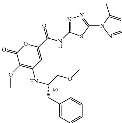
5-methoxy-4-([(2S)-1-methoxy-3-phenylpropan-2-yl]amino)-N-[5-(5-methylpyrazol-1-yl)-1,3,4-thiadiazol-2-yl]-6-oxopyran-2-carboxamide
