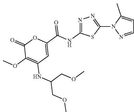
Compound 10 4-((1,3-dimethoxypropan-2-yl)amino)-3-methoxy-N-(5-(5-methyl-1H-pyrazol-1-yl)-1,3,4-thiadiazol-2-yl)-2-oxo-2H-pyran-6-carboxamide
