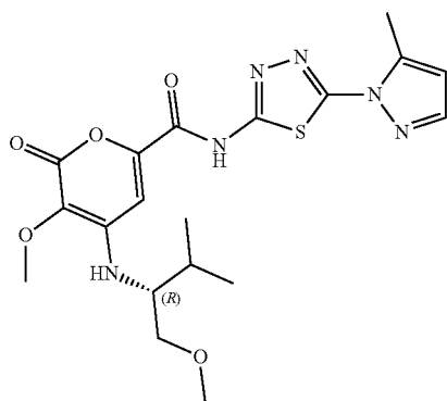
(R)-3-methoxy-4-((1-methoxy-3-methylbutan-2-yl)amino)-N-(5-(5-methyl-1H-pyrazol-1-yl)-1,3,4-thiadiazol-2-yl)-2-oxo-2H-pyran-6-carboxamide
