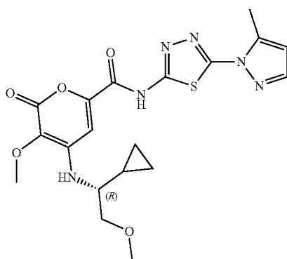
(R)-4-((1-cyclopropyl-2-methoxyethyl)amino)-3-methoxy-N-(5-(5-methyl-1H-pyrazol-1-yl)-1,3,4-thiadiazol-2-yl)-2-oxo-2H-pyran-6-carboxamide
