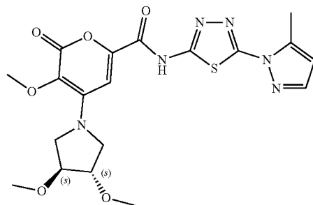
4-((3S,4S)-3,4-dimethoxypyrrolidin-1-yl)-3-methoxy-N-(5-(5-methyl-1H-pyrazol-1-yl)-1,3,4-thiadiazol-2-yl)-2-oxo-2H-pyran-6-carboxamide
