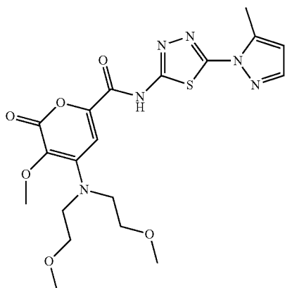
4-(bis(2-methoxyethyl)amino)-3-methoxy-N-(5-(5-methyl-1H-pyrazol-1-yl)-1,3,4-thiadiazol-2-yl)-2-oxo-2H-pyran-6-carboxamide
