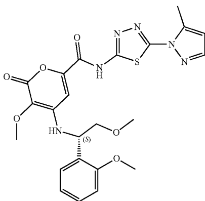
(S)-3-methoxy-4-((2-methoxy-1-(2-methoxyphenyl)ethyl)amino)-N-(5-(5-methyl-1H-pyrazol-1-yl)-1,3,4-thiadiazol-2-yl)-2-oxo-2H-pyran-6-carboxamide
