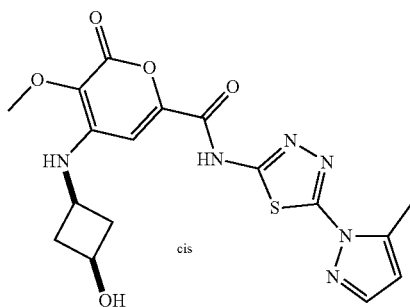
4-(((1,3-cis)-3-hydroxycyclobutyl)amino)-3-methoxy-N-(5-(5-methyl-1H-pyrazol-1-yl)-1,3,4-thiadiazol-2-yl)-2-oxo-2H-pyran-6-carboxamide
