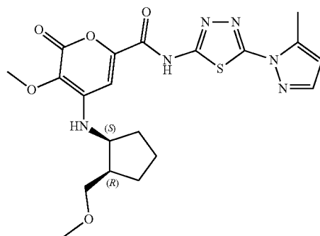
3-methoxy-4-(((1S,2R)-2-(methoxymethyl)cyclopentyl)amino)-N-(5-(5-methyl-1H-pyrazol-1-yl)-1,3,4-thiadiazol-2-yl)-2-oxo-2H-pyran-6-carboxamide
