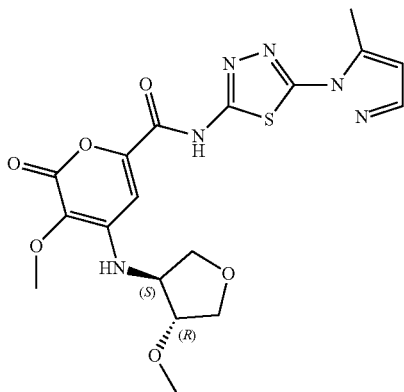
3-methoxy-4-(((3S,4R)-4-methoxytetrahydrofuran-3-yl)amino)-N-(5-(5-methyl-1H-pyrazol-1-yl)-1,3,4-thiadiazol-2-yl)-2-oxo-2H-pyran-6-carboxamide
