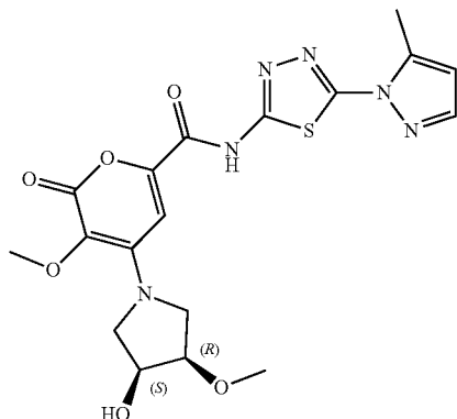
4-((3S,4R)-3-hydroxy-4-methoxypyrrolidin-1-yl)-3-methoxy-N-(5-(5-methyl-1H-pyrazol-1-yl)-1,3,4-thiadiazol-2-yl)-2-oxo-2H-pyran-6-carboxamide
