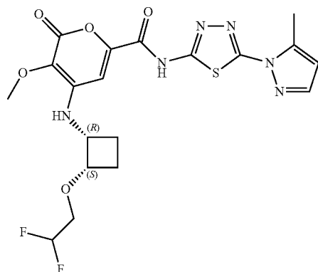
Compound 173* 4-(((1R,2S)-2-(2,2-difluoroethoxy)cyclobutyl)amino)-3-methoxy-N-(5-(5-methyl-1H-pyrazol-1-yl)-1,3,4-thiadiazol-2-yl)-2-oxo-2H-pyran-6-carboxamide
