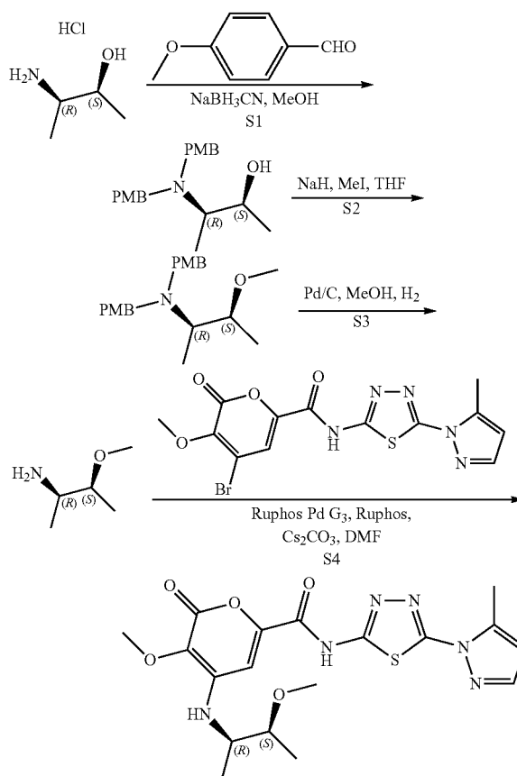
Compound 166 3-methoxy-4-(((2R,3S)-3-methoxybutan-2-yl)amino)-N-(5-(5-methyl-1H-pyrazol-1-yl)-1,3,4-thiadiazol-2-yl)-2-oxo-2H-pyran-6-carboxamide
