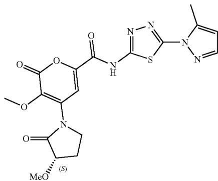
5-methoxy-4-[(3S)-3-methoxy-2-oxopyrrolidin-1-yl]-N-[5-(5- methylpyrazol-1-yl)-1,3,4-thiadiazol-2-yl]-6-oxopyran-2-carboxamide
