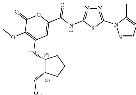
4-(((1R,2S)-2-(hydroxymethyl)cyclopentyl)amino)-3-methoxy-N-(5-(5-methyl-1H-pyrazol-1-yl)-1,3,4-thiadiazol-2-yl)-2-oxo-2H-pyran-6-carboxamide
