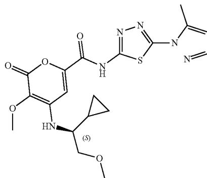
(S)-4-((1-cyclopropyl-2-methoxyethyl)amino)-3-methoxy-N-(5-(5-methyl-1H-pyrazol-1-yl)-1,3,4-thiadiazol-2-yl)-2-oxo-2H-pyran-6-carboxamide
