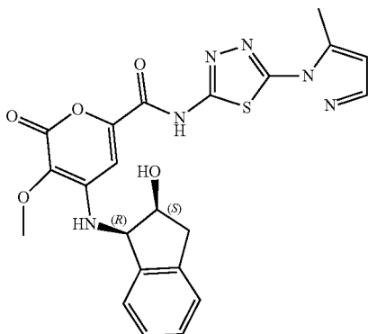
4-(((1R,2S)-2-hydroxy-2,3-dihydro-1H-inden-1-yl)amino)-3-methoxy-N-(5-(5-methyl-1H-pyrazol-1-yl)-1,3,4-thiadiazol-2-yl)-2-oxo-2H-pyran-6-carboxamide
