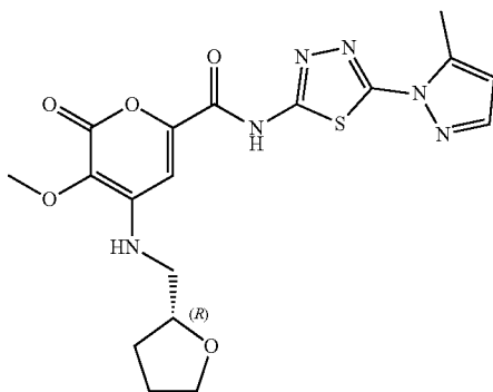
(R)-3-methoxy-N-(5-(5-methyl-1H-pyrazol-1-yl)-1,3,4-thiadiazol-2-yl)-2-oxo-4-(((tetrahydrofuran-2-yl)methyl)amino)-2H-pyran-6-carboxamide
