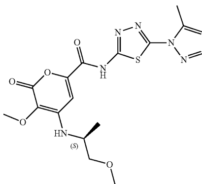
(S)-3-methoxy-4-((1-methoxypropan-2-yl)amino)-N-(5-(5-methyl-1H-pyrazol-1-yl)-1,3,4-thiadiazol-2-yl)-2-oxo-2H-pyran-6-carboxamide
