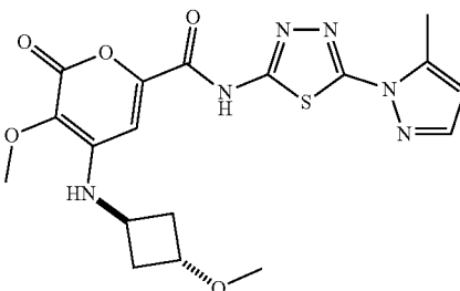
3-methoxy-4-(((1,3-trans)-3-methoxycyclobutyl)amino)-N-(5-(5-methyl-1H-pyrazol-1-yl)-1,3,4-thiadiazol-2-yl)-2-oxo-2H-pyran-6-carboxamide
