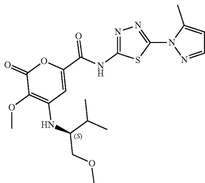
(S)-3-methoxy-4-((1-methoxy-3-methylbutan-2-yl)amino)-N-(5-(5-methyl-1H-pyrazol-1-yl)-1,3,4-thiadiazol-2-yl)-2-oxo-2H-pyran-6-carboxamide
