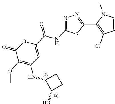
N-(5-(3-chloro-1-methyl-1H-pyrrol-2-yl)-1,3,4-thiadiazol-2-yl)-4-(((1R,2S)-2-hydroxycyclobutyl)amino)-3-methoxy-2-oxo-2H-pyran-6-carboxamide
