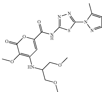
4-((1,3-dimethoxypropan-2-yl)amino)-3-methoxy-N-(5-(5-methyl-1H-pyrazol-1-yl)-1,3,4-thiadiazol-2-yl)-2-oxo-2H-pyran-6-carboxamide
