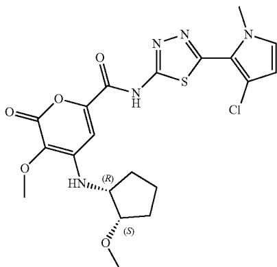
N-(5-(3-chloro-1-methyl-1H-pyrrol-2-yl)-1,3,4-thiadiazol-2-yl)-3-methoxy-4-(((1R,2S)-2-methoxycyclopentyl)amino)-2-oxo-2H-pyran-6-carboxamide
