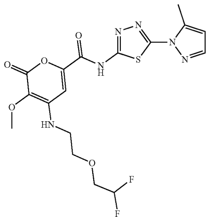
4-((2-(2,2-difluoroethoxy)ethyl)amino)-3-methoxy-N-(5-(5-methyl-1H-pyrazol-1-yl)-1,3,4-thiadiazol-2-yl)-2-oxo-2H-pyran-6-carboxamide
