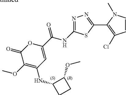
Compound 133* N-(5-(3-chloro-1-methyl-1H-pyrrol-2-yl)-1,3,4-thiadiazol-2-yl)-3-methoxy-4-(((1S,2R)-2-methoxycyclobutyl)amino)-2-oxo-2H-pyran-6-carboxamide
