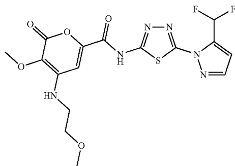
N-(5-(5-(difluoromethyl)-1H-pyrazol-1-yl)-1,3,4-thiadiazol-2-yl)-3-methoxy-4-((2-methoxyethyl)amino)-2-oxo-2H-pyran-6-carboxamide
