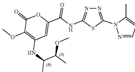
5-methoxy-4-([(2R,3S)-3-methoxybutan-2-yl]amino)-N-[5-(5-methylpyrazol-1-yl)-1,3,4-thiadiazol-2-yl]-6-oxopyran-2-carboxamide
