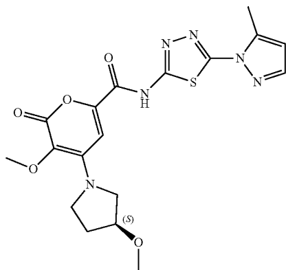
(S)-3-methoxy-4-(3-methoxypyrrolidin-1-yl)-N-(5-(5-methyl-1H-pyrazol-1-yl)-1,3,4-thiadiazol-2-yl)-2-oxo-2H-pyran-6-carboxamide
