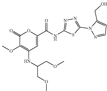
4-((1,3-dimethoxypropan-2-yl)amino)-N-(5-(5-(hydroxymethyl)-1H-pyrazol-1-yl)-1,3,4-thiadiazol-2-yl)-3-methoxy-2-oxo-2H-pyran-6-carboxamide
