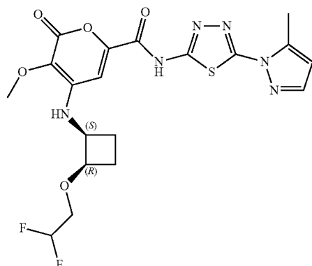
Compound 172* 4-(((1S,2R)-2-(2,2-difluoroethoxy)cyclobutyl)amino)-3-methoxy-N-(5-(5-methyl-1H-pyrazol-1-yl)-1,3,4-thiadiazol-2-yl)-2-oxo-2H-pyran-6-carboxamide
