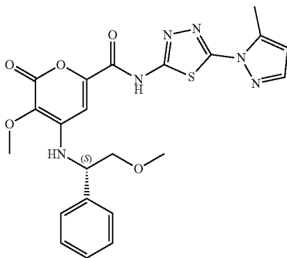
(S)-3-methoxy-4-((2-methoxy-1-phenylethyl)amino)-N-(5-(5-methyl-1H-pyrazol-1-yl)-1,3,4-thiadiazol-2-yl)-2-oxo-2H-pyran-6-carboxamide
