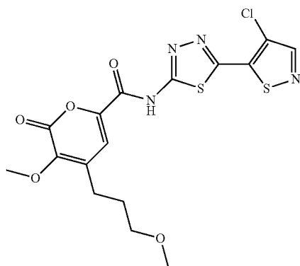
Compound 139 N-(5-(4-chloroisothiazol-5-yl)-1,3,4-thiadiazol-2-yl)-3-methoxy-4-((2-methoxyethyl)amino)-2-oxo-2H-pyran-6-carboxamide
