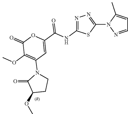
5-methoxy-4-[(3R)-3-methoxy-2-oxopyrrolidin-1-yl]-N-[5-(5- methylpyrazol-1-yl)-1,3,4-thiadiazol-2-yl]-6-oxopyran-2-carboxamide
