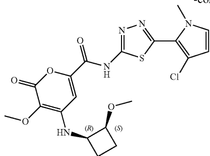
Compound 132* N-(5-(3-chloro-1-methyl-1H-pyrrol-2-yl)-1,3,4-thiadiazol-2-yl)-3-methoxy-4-(((1R,2S)-2-methoxycyclobutyl)amino)-2-oxo-2H-pyran-6-carboxamide
