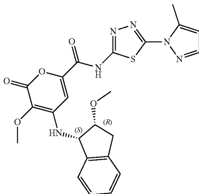
3-methoxy-4-(((1S,2R)-2-methoxy-2,3-dihydro-1H-inden-1-yl)amino)-N-(5-(5-methyl-1H-pyrazol-1-yl)-1,3,4-thiadiazol-2-yl)-2-oxo-2H-pyran-6-carboxamide
