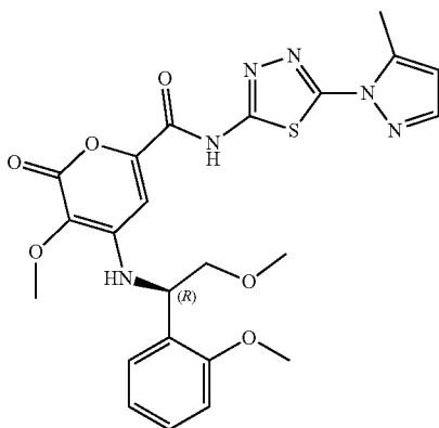
(R)-3-methoxy-4-((2-methoxy-1-(2-methoxyphenyl)ethyl)amino)-N-(5-(5-methyl-1H-pyrazol-1-yl)-1,3,4-thiadiazol-2-yl)-2-oxo-2H-pyran-6-carboxamide
