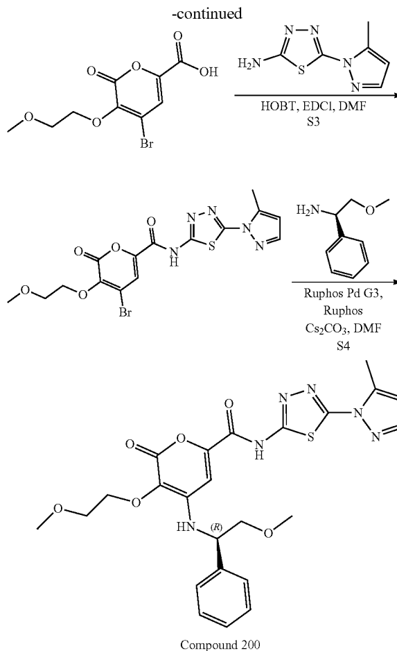
Compound 200 (R)-4-((2-methoxy-1-phenylethyl)amino)-3-(2-methoxyethoxy)-N-(5-(S-methyl-1H-pyrazol-1-yl)-1,3,4-thiadiazol-2-yl)-2-oxo-2H-pyran-6-carboxamide
