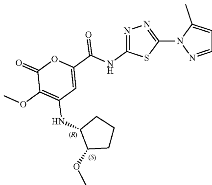
3-methoxy-4-(((1S,2R)-2-methoxycyclopentyl)amino)-N-(5-(5-methyl-1H-pyrazol-1-yl)-1,3,4-thiadiazol-2-yl)-2-oxo-2H-pyran-6-carboxamide
