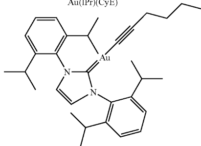
Au(IPr)(n-BuE)
