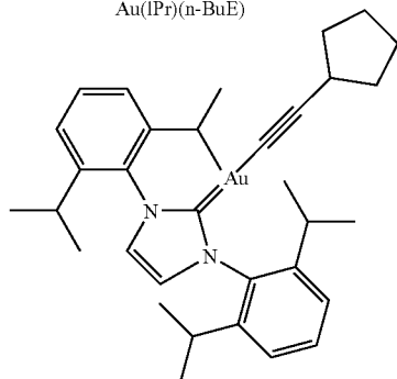
Au(IPr)(CpE)
