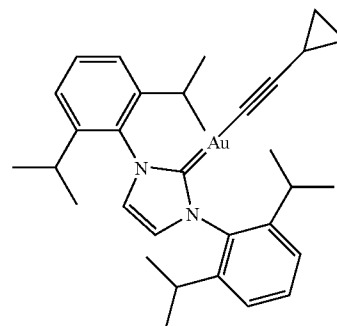
Au(IPr)(cPrE)
