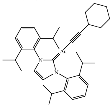
Au(IPr)(CyE)
