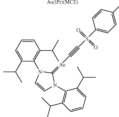
Au(IPr)(pTsE)
