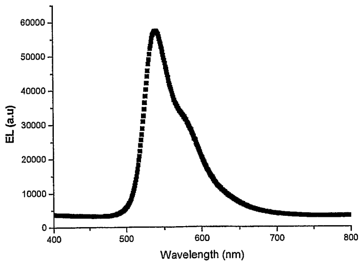
EL spectrum
