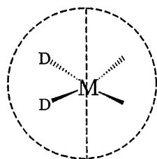
cis
