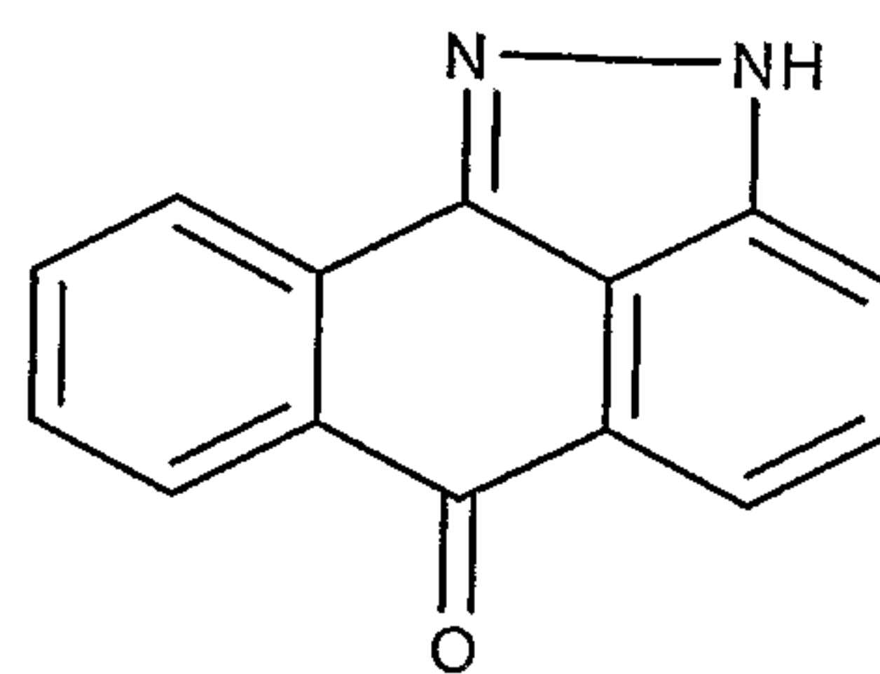
2 H -Dibenzo[ cd,g ] indazol-6-one ;
