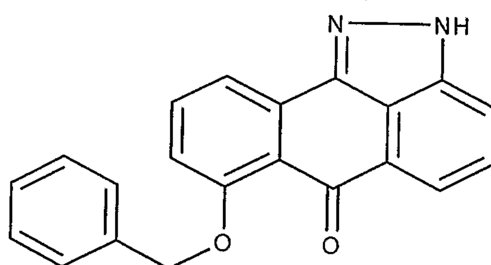
7-Benzyloxy-2 H -dibenzo[ cd,g ]indazol- 6-one ;
