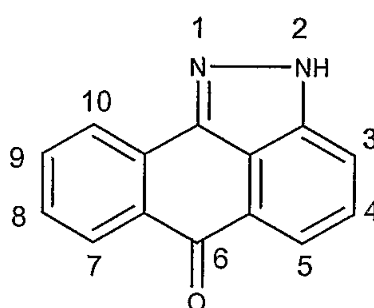
2 H -Dibenzo[ cd,g ]indazol-6-one (IIIF)
