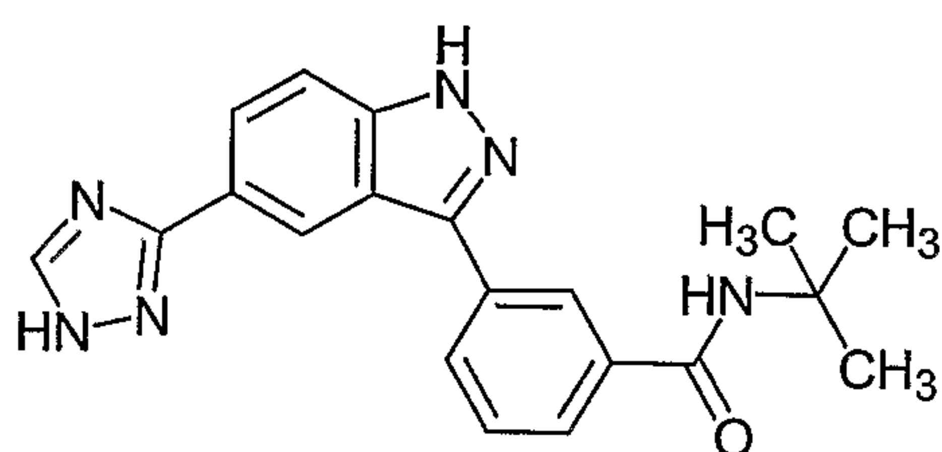
N -tert-Butyl-3-[5-(1 H -[1,2,4]triazol-3-yl)-1 H -indazol-3-yl]-benzamide ;
