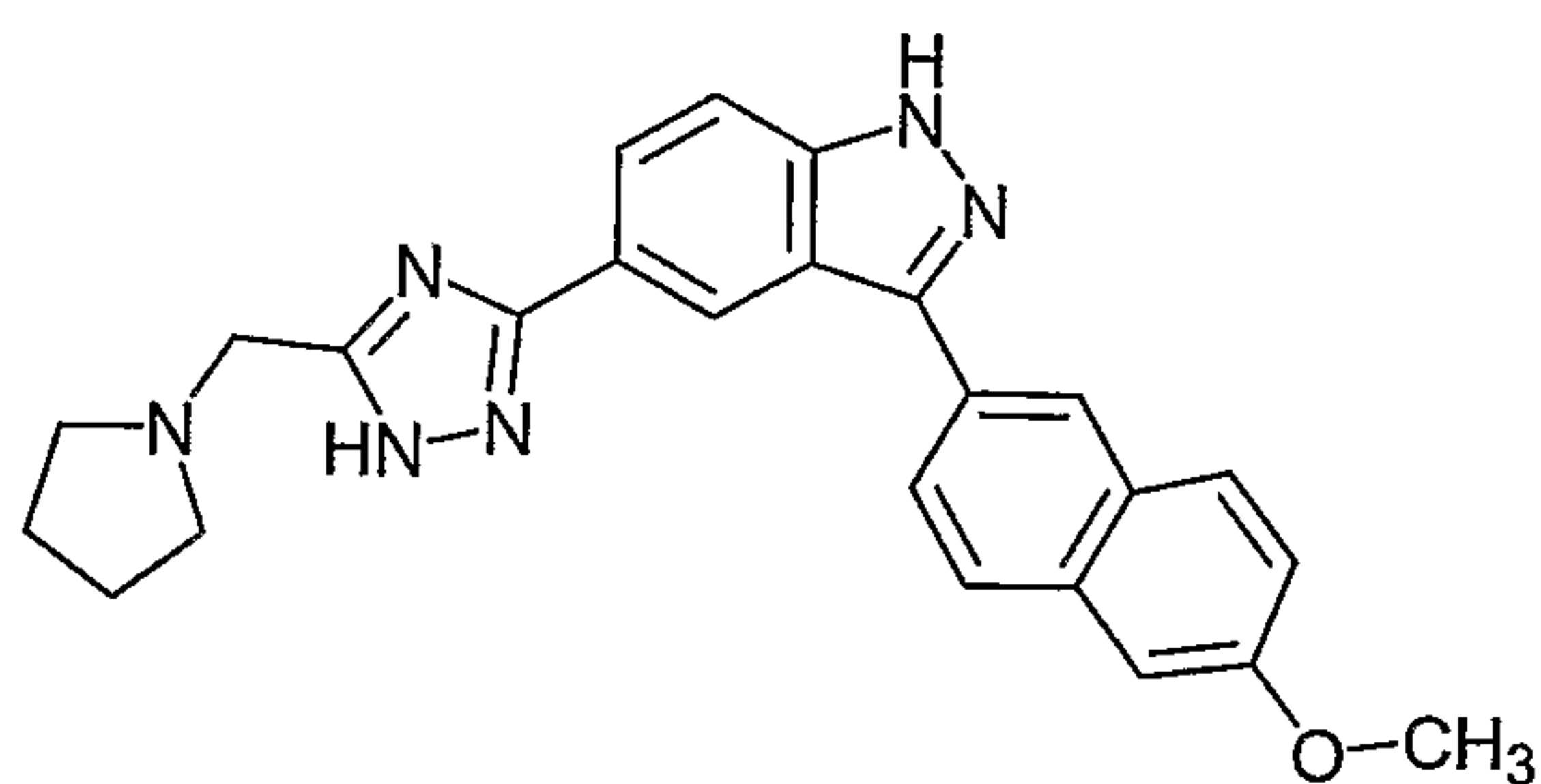
3-(6-Methoxy-naphthalen-2-yl)-5-(5-pyrrolidin-1-ylmethyl- 1H\text{-}[1,2,4]\text{triazol-}3\text{-yl}) - 1H -indazole ;
