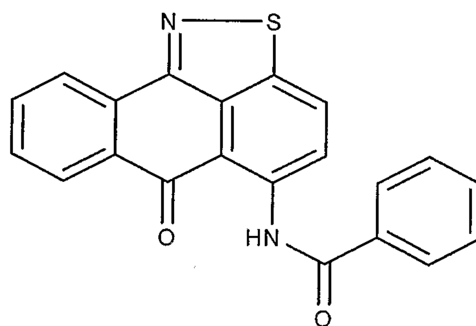
N -(6-Oxo-6 H -anthra[9,1- cd ]isothiazol-5- yl)-benzamide ;
