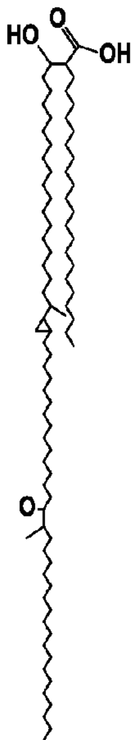
Keto
