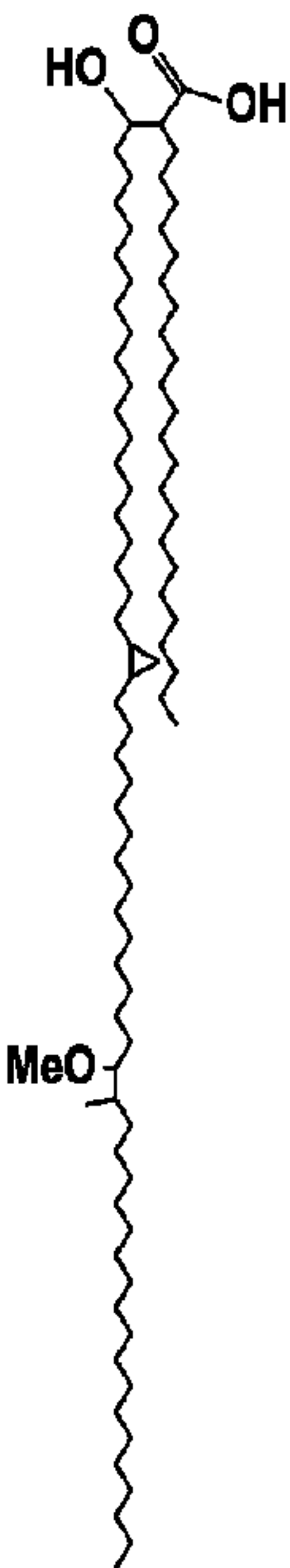
Methoxy
