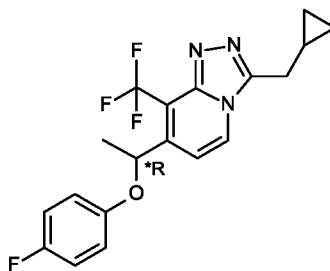
Сполука 2-b
