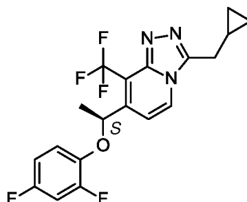
Сполука 6-b
