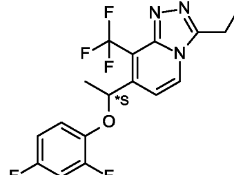
Сполука 27-b
