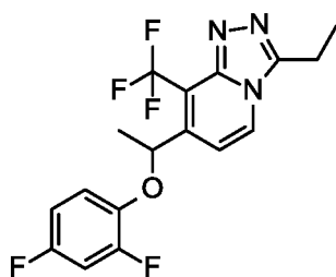
Сполука 24-b
