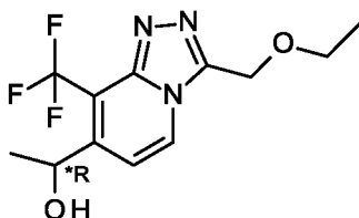
Проміжна сполука 24b
