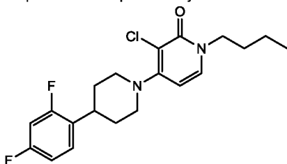
(спол. № 25-a)
