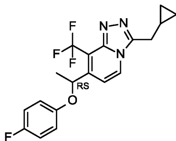
Сполука 1-b
