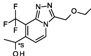
Проміжна сполука 24c
