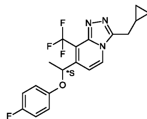
Сполука 3-b
