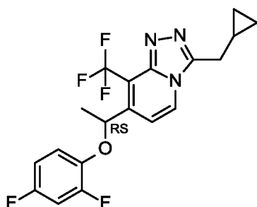
Сполука 4-b
