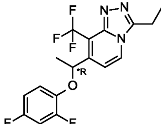
Сполука 26-b
