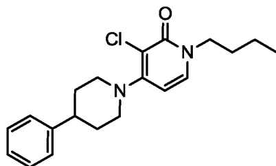
(спол. № 2-a)
