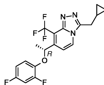
Сполука 5-b
