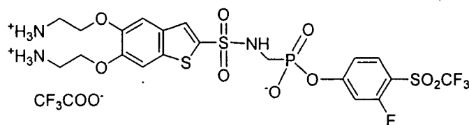
3-fluoro-4-[(trifluoromethyl)sulfonyl]phenyl-[({[5,6-bis(2-ammonioethoxy)-1-benzothien-2-yl]-sulfonyl}amino)methyl]phosphonate trifluoroacetate
